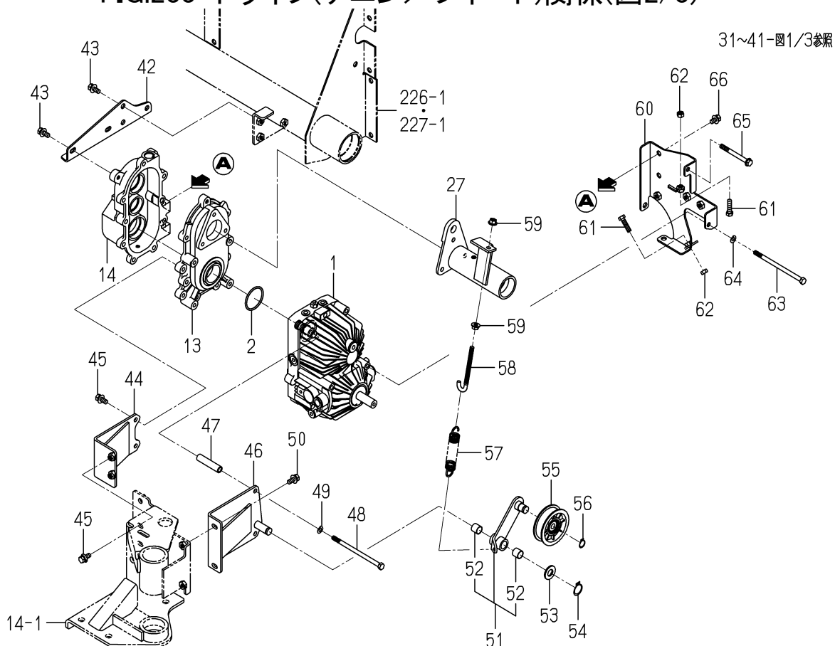
FIG.233 ドライブ(チェン/フイード)関係(図2/3)
