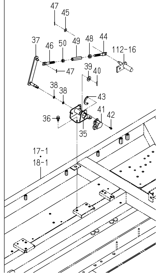
FIG. 77 センサ(ソウコウ)関係(図2/2)
