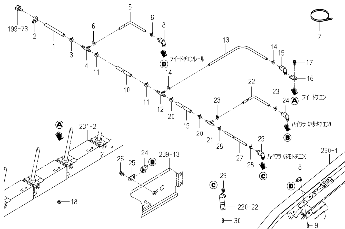
FIG.202 ノズル(オイリング／ダツコク)関係
