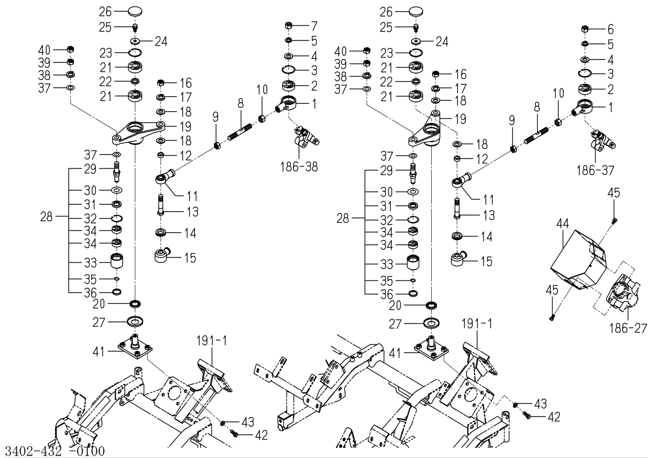
FIG.140 ドライブ(カリハ)関係
