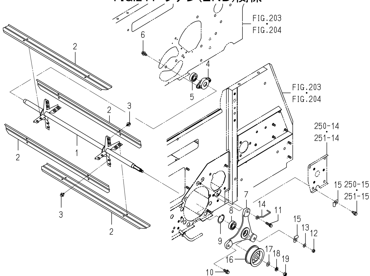
FIG.244 ファン(2ND)関係
