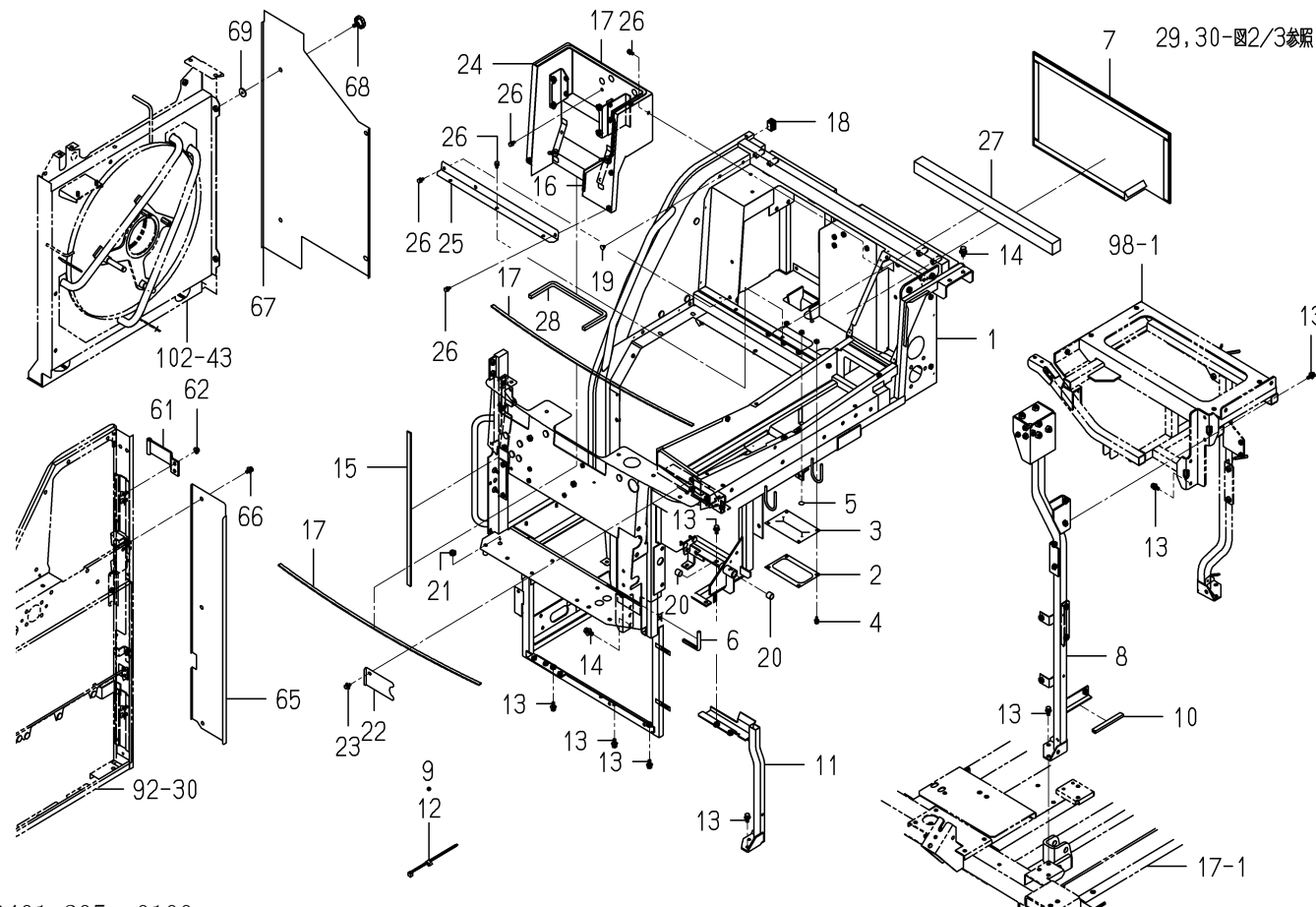
FIG. 30 フレーム(コントロール)関係(ZC型除く)(図1/3)
