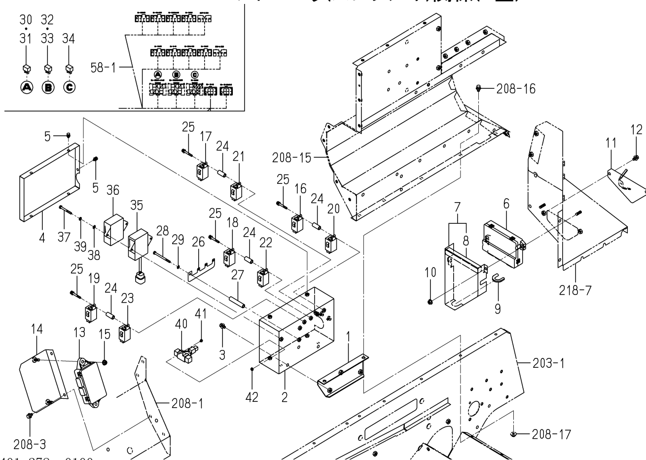
FIG. 73 コントローラ(スレッツシヤ)関係(Z型)
