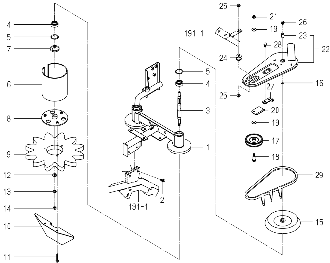
FIG.142 レイクアツプ(LH／2ND, 3RD)関係(図1/2)
