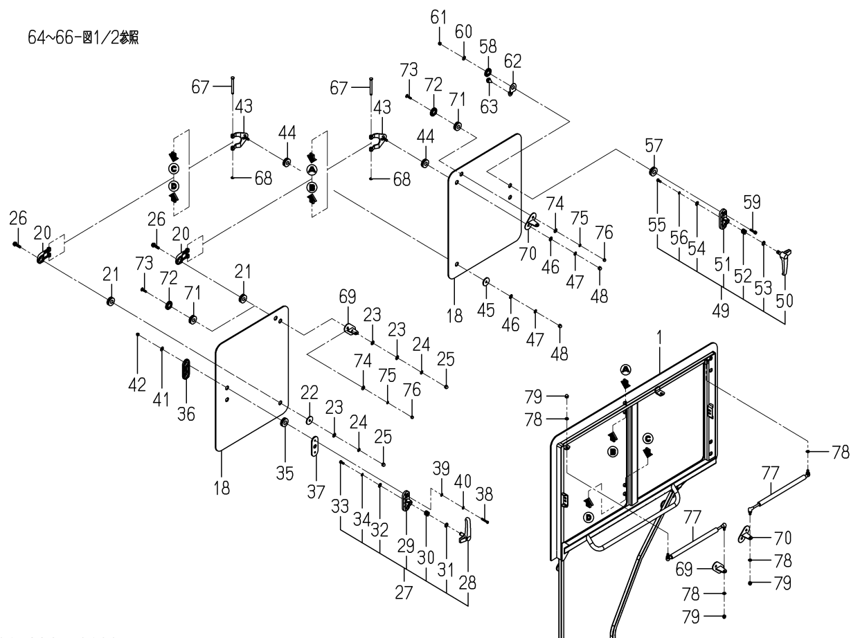
FIG. 47 ドア(キャビン)関係(ZC型)(図2/2)
