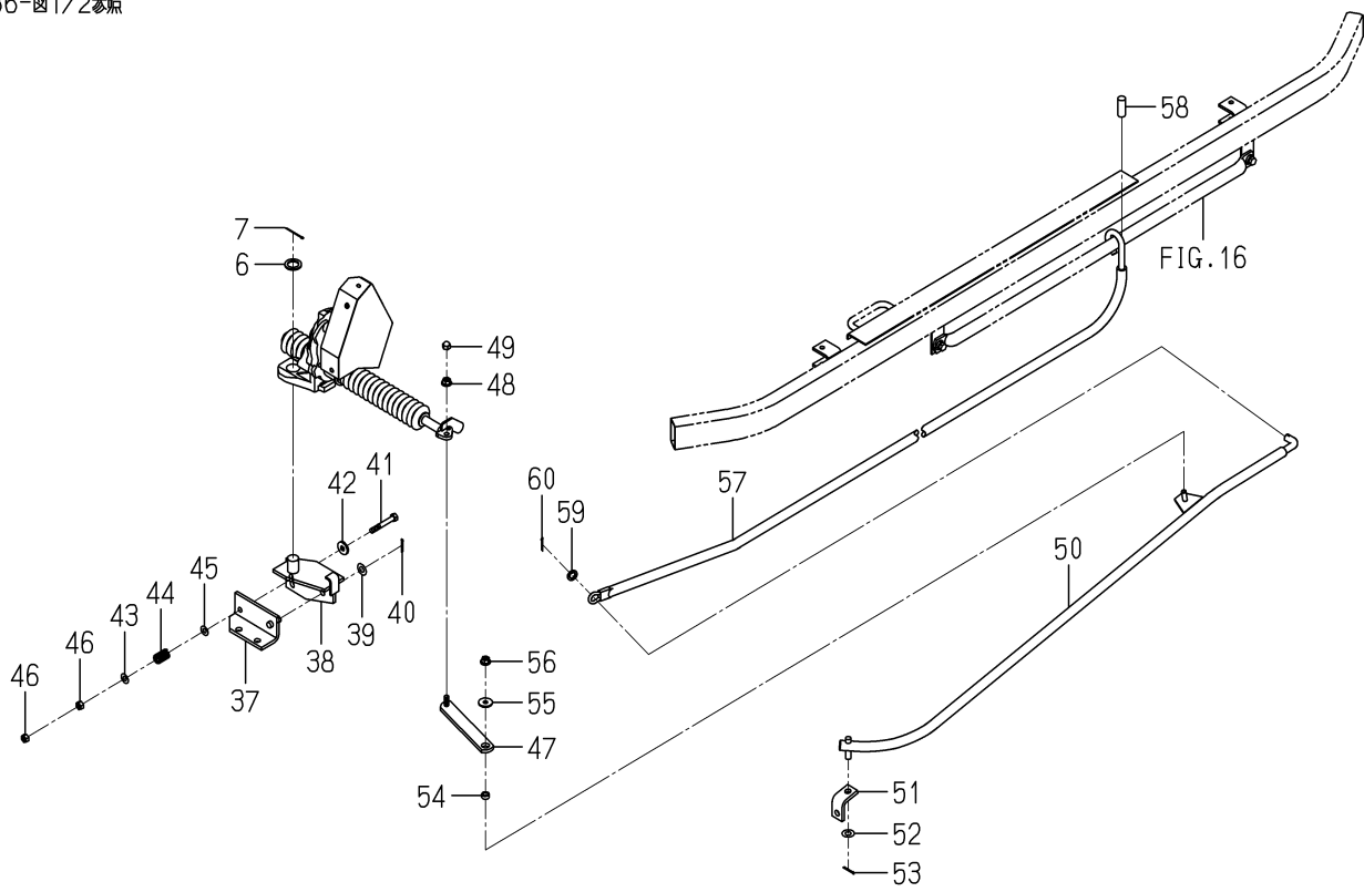
FIG.122 ガイド(ナロー／LH)関係(図2/2)
