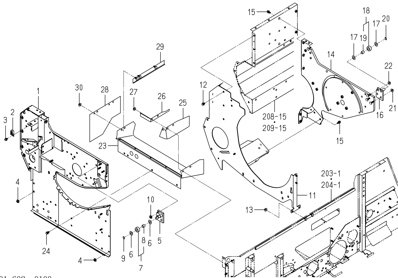
FIG.205 ホンタイ(2)関係
