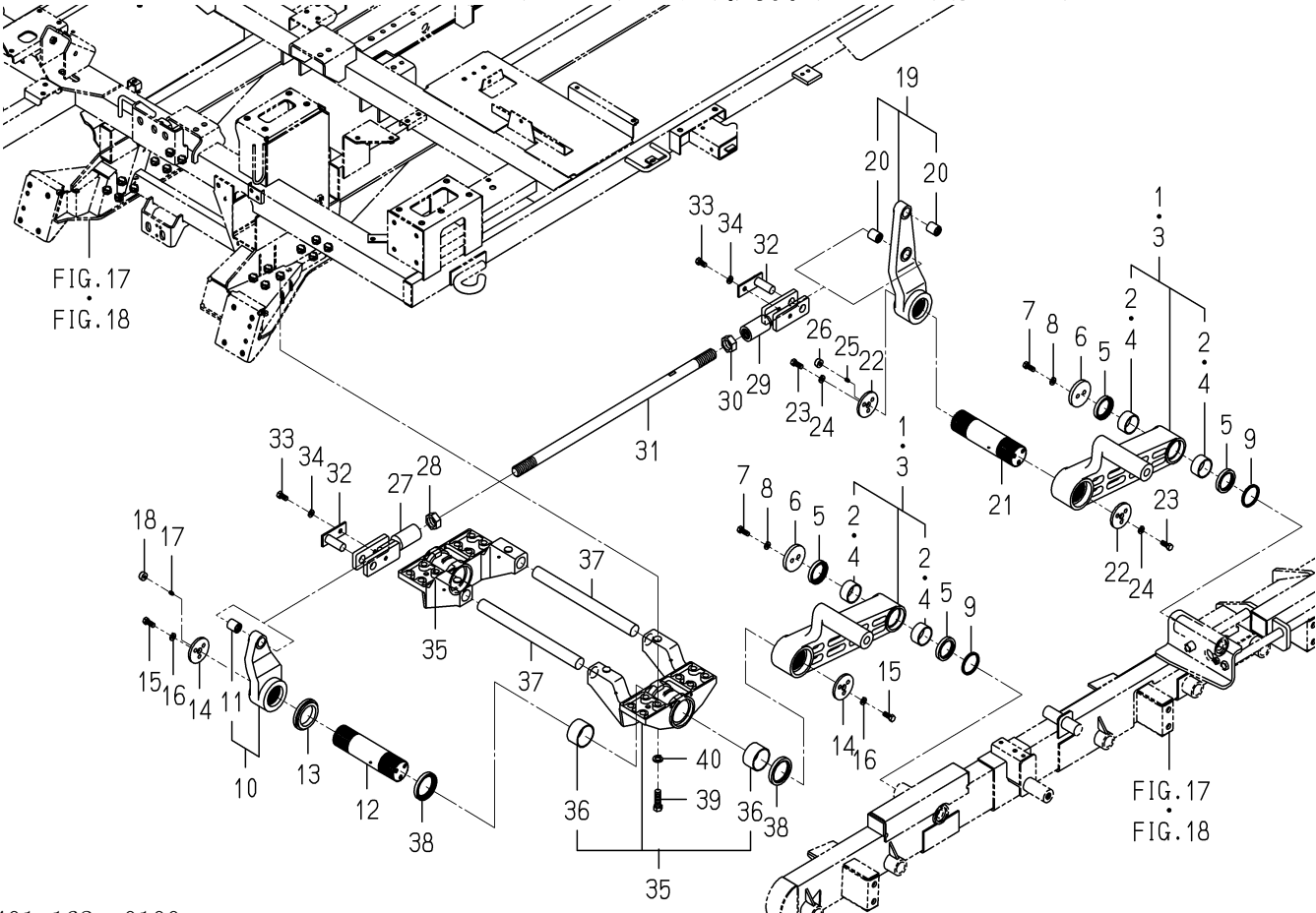
FIG. 19 アーム(ローリング)関係(LW型)(図1/2)
