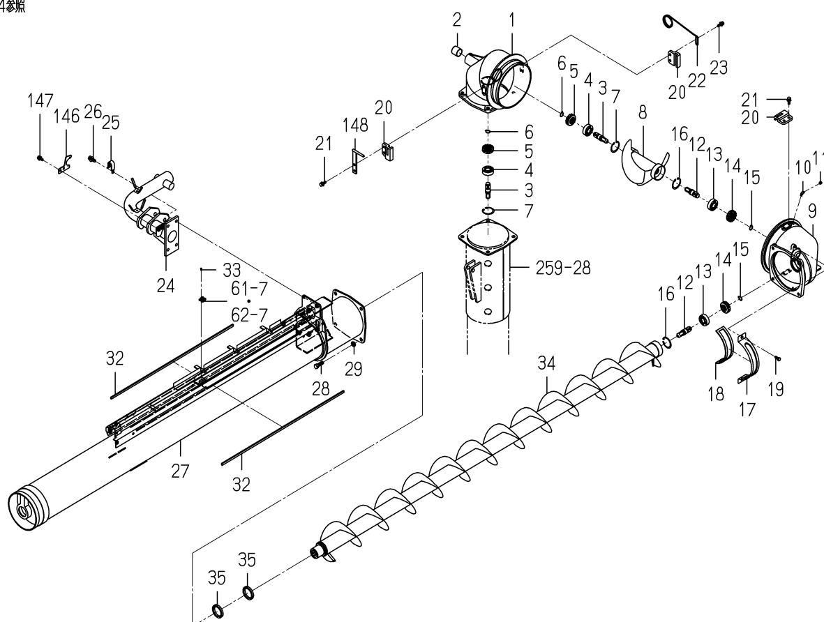
FIG.260 ドライブ(オーガ/スイング)関係(Z型)(図1/4)
