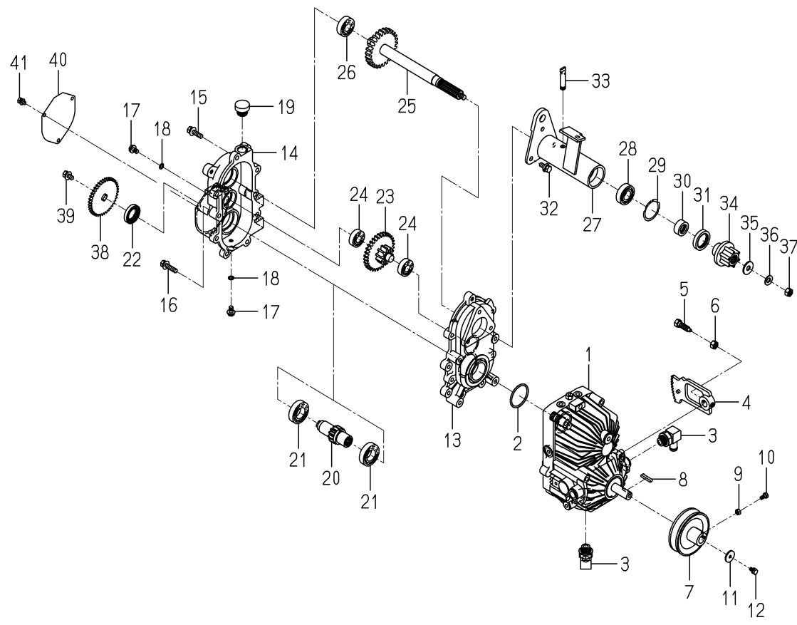
FIG.233 ドライブ(チェン／フイード)関係(図1/3)
