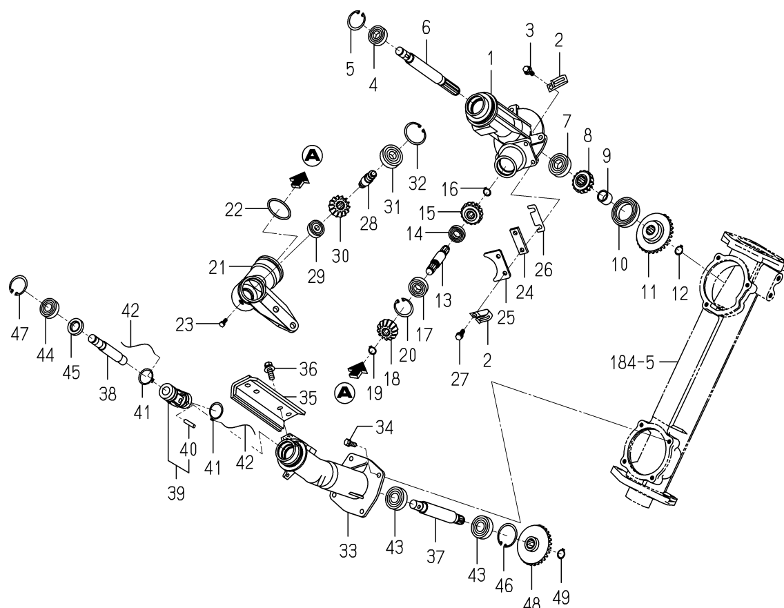
FIG.185 ケース(ギヤー／ネモト／RH／センタ)関係
