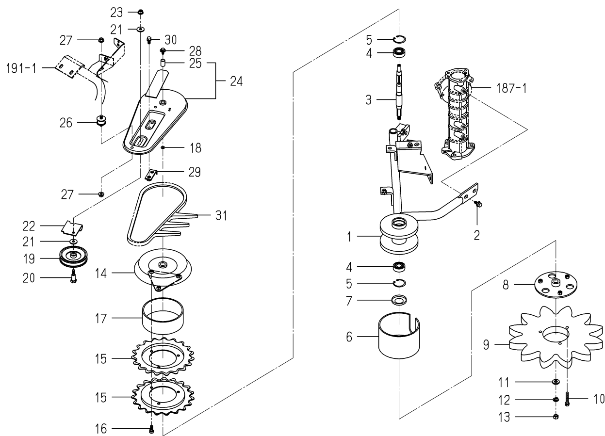
FIG.141 レイクアップ(LH/1ST)関係
