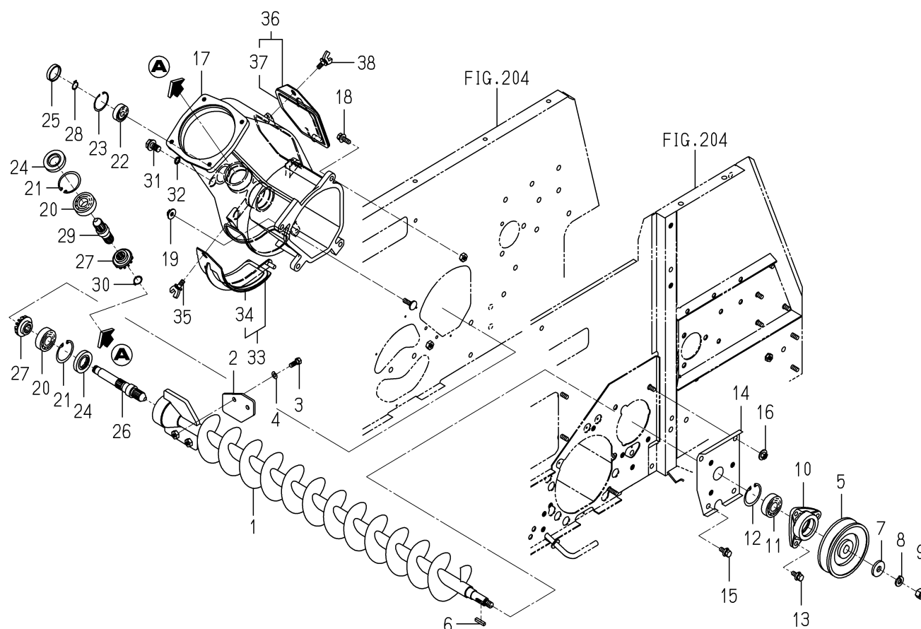
FIG.251 スパイラル(2ND)関係(T型)
