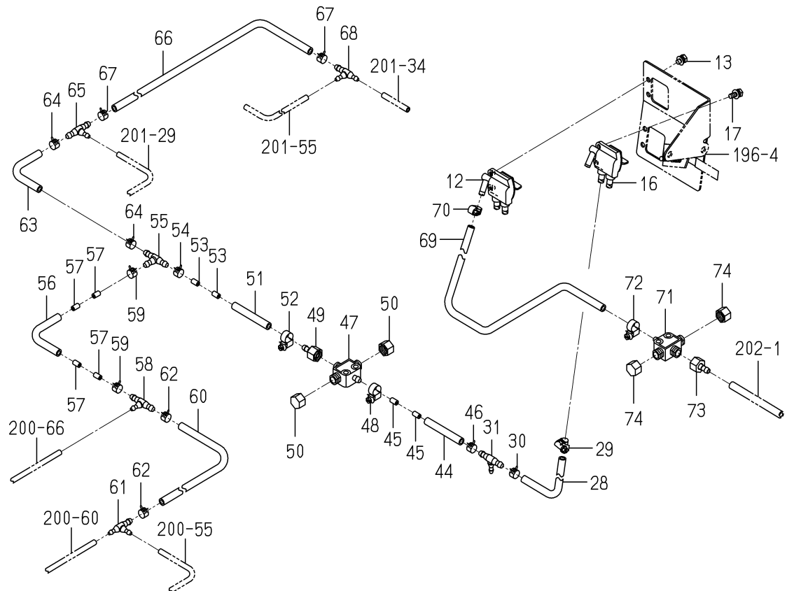
FIG.199 パイピング(オイリング)関係(図2/2)
