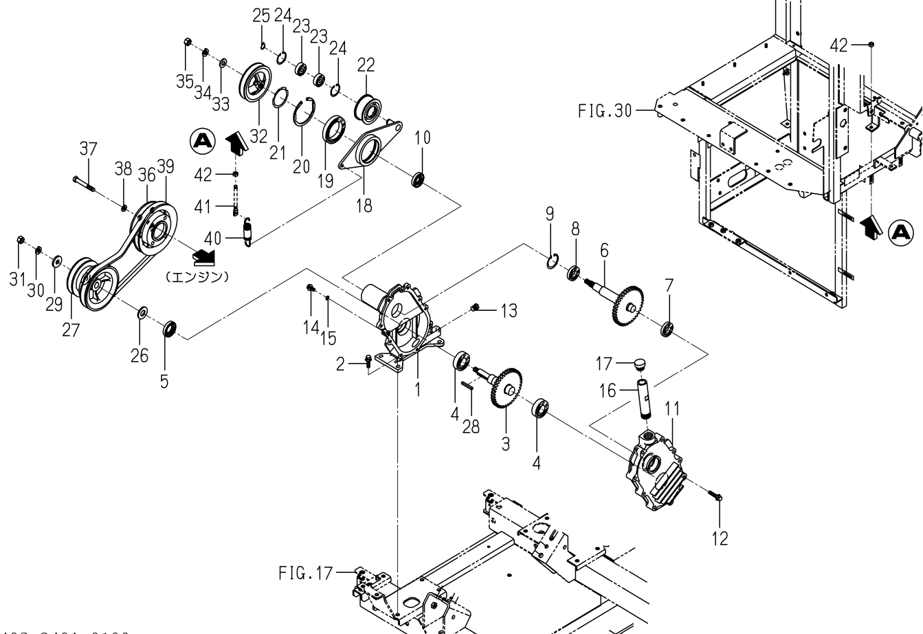
FIG.102 ファン(リバー)関係(ZC型除く)(図1/3)
