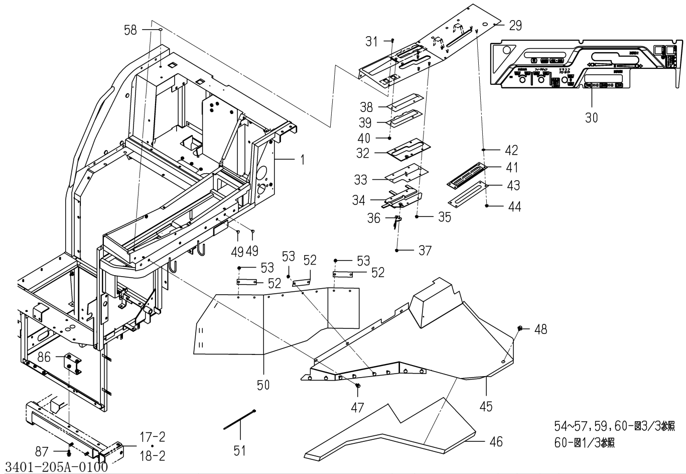
FIG. 31 フレーム(コントロール)関係(ZC型)(図2/3)
