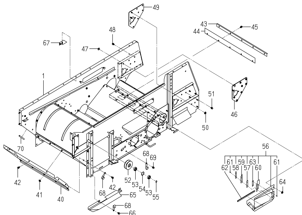
FIG.203 ホンタイ(1)関係(Z型)(図2/2)
