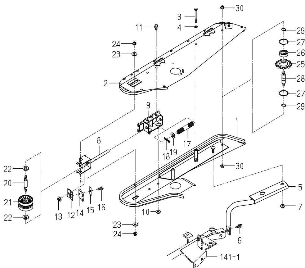
FIG.172 ケース(ホサキ/LH)関係
