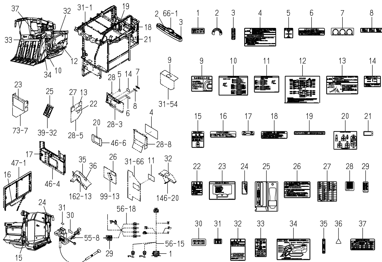
FIG.276 ラベル(コントロール, コーシヨン)(C型)(図1/2)
