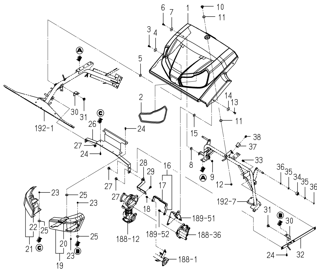
FIG.197 カバー(ダスト)関係(ZC型除く)(図1/2)
