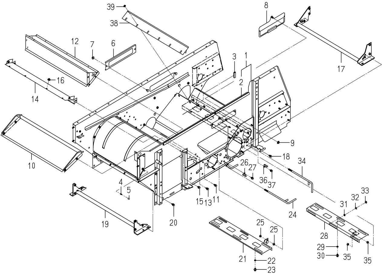
FIG.203 ホンタイ(1)関係(Z型)(図1/2)
