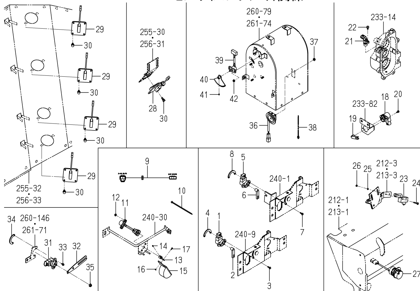
FIG. 79 センサ(スレッシヤ)関係
