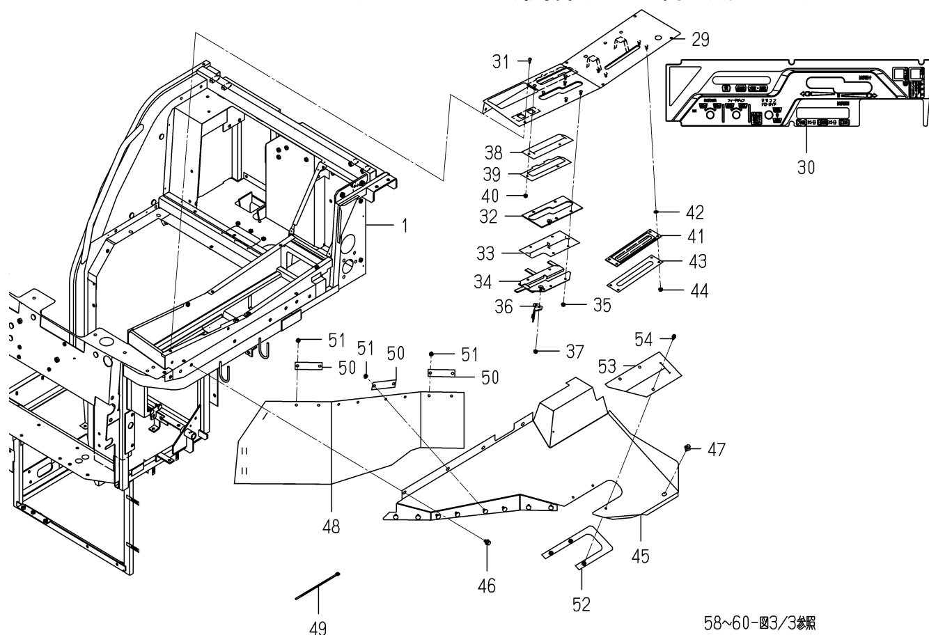
FIG. 30 フレーム(コントロール)関係(ZC型除く)(図2/3)
