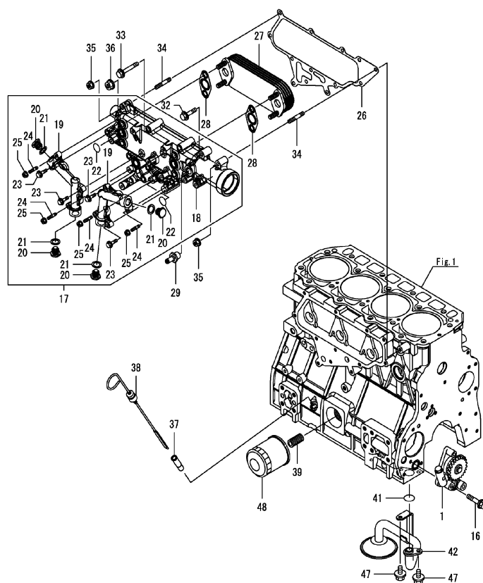
FIG.011 潤滑油システム(SISC2型)
