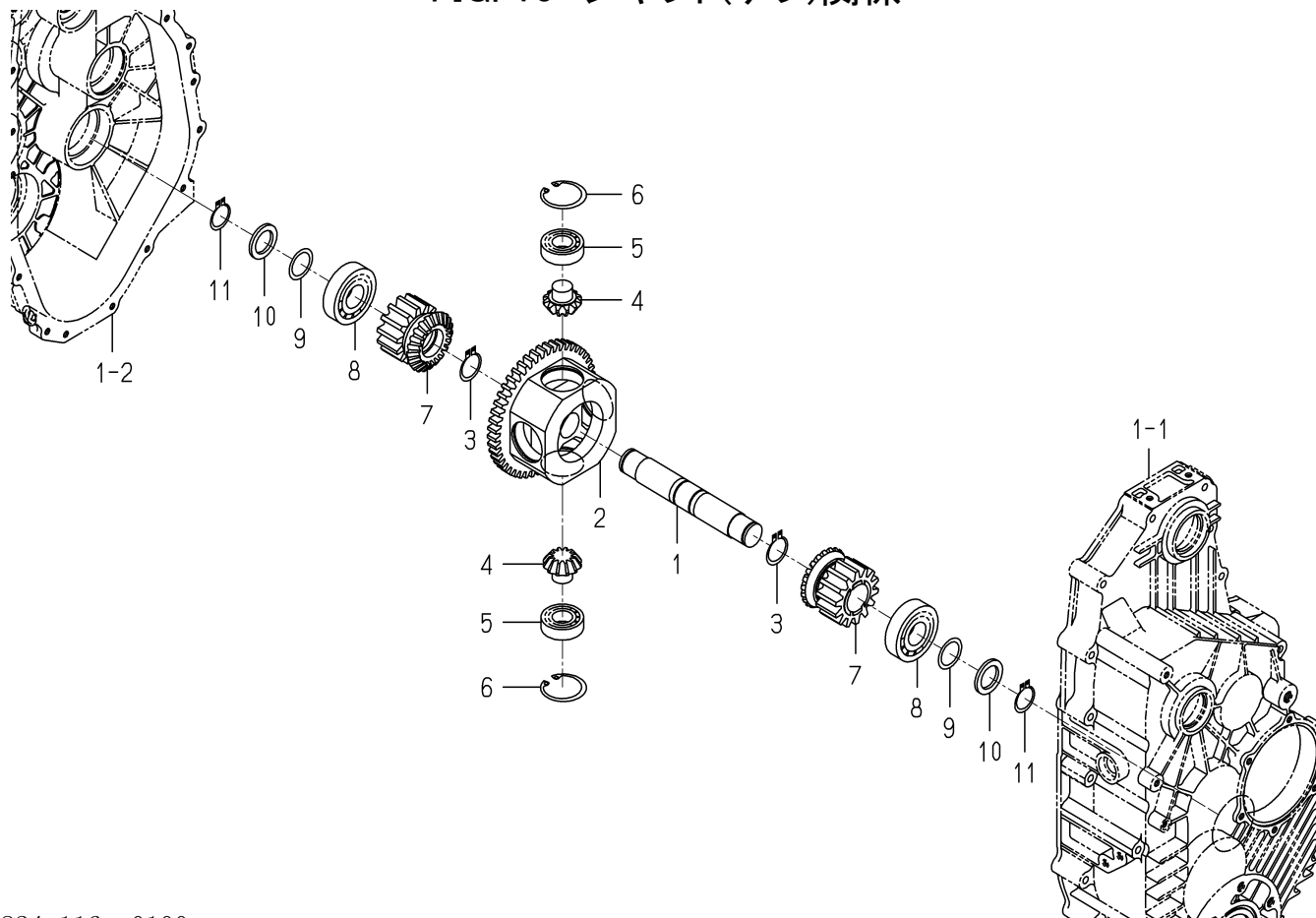
FIG. 10 シャフト(デフ)関係
