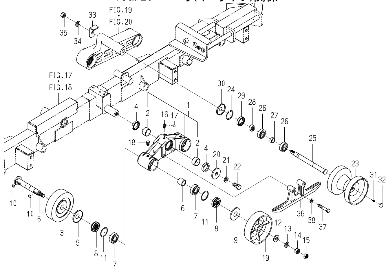
FIG. 23 ローラ(イコライザ)関係
