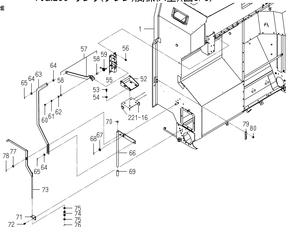
FIG.255 タンク(グレン)関係(A型)(図3/3)
