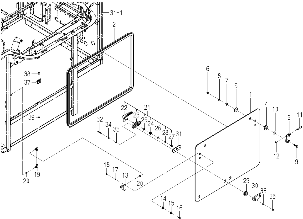
FIG. 49 ウインド(LH／キャビン)関係(ZC型)
