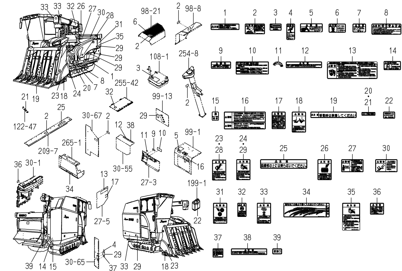
FIG.268 ラベル(コーション)(T型)
