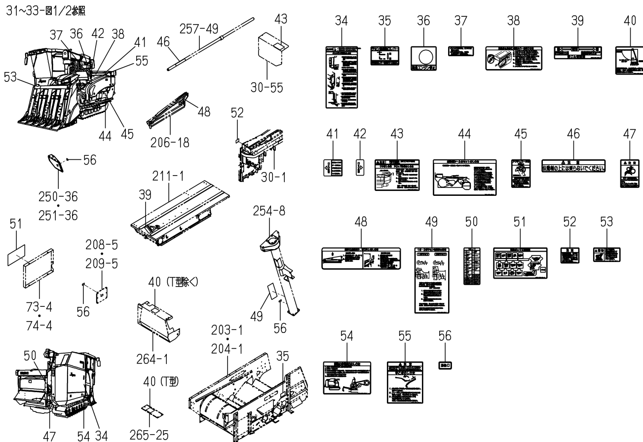
FIG.275 ラベル(コントロール, コーシヨン)(ZC型除く)(図2/2)
