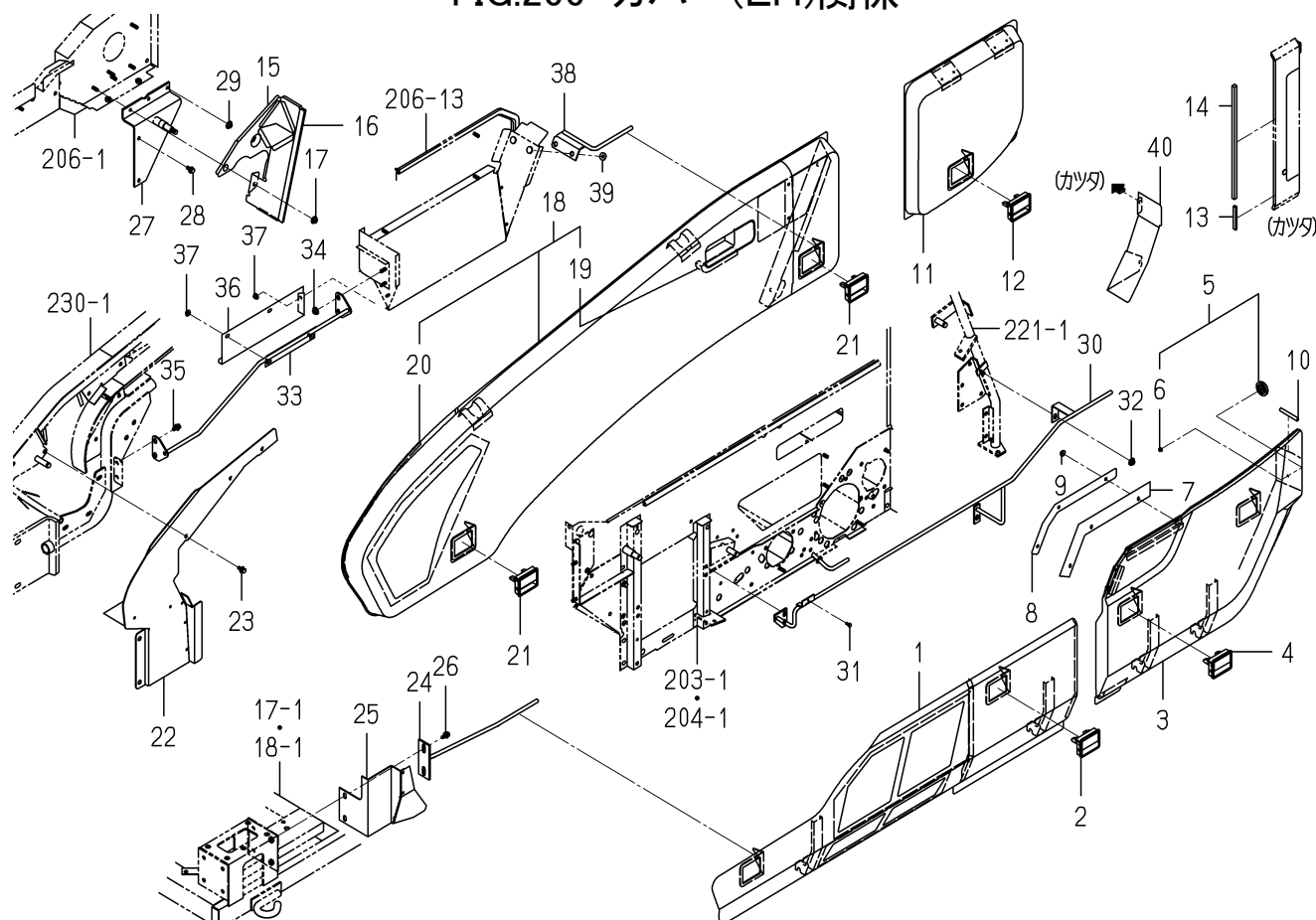
FIG.266 カバー(LH)関係
