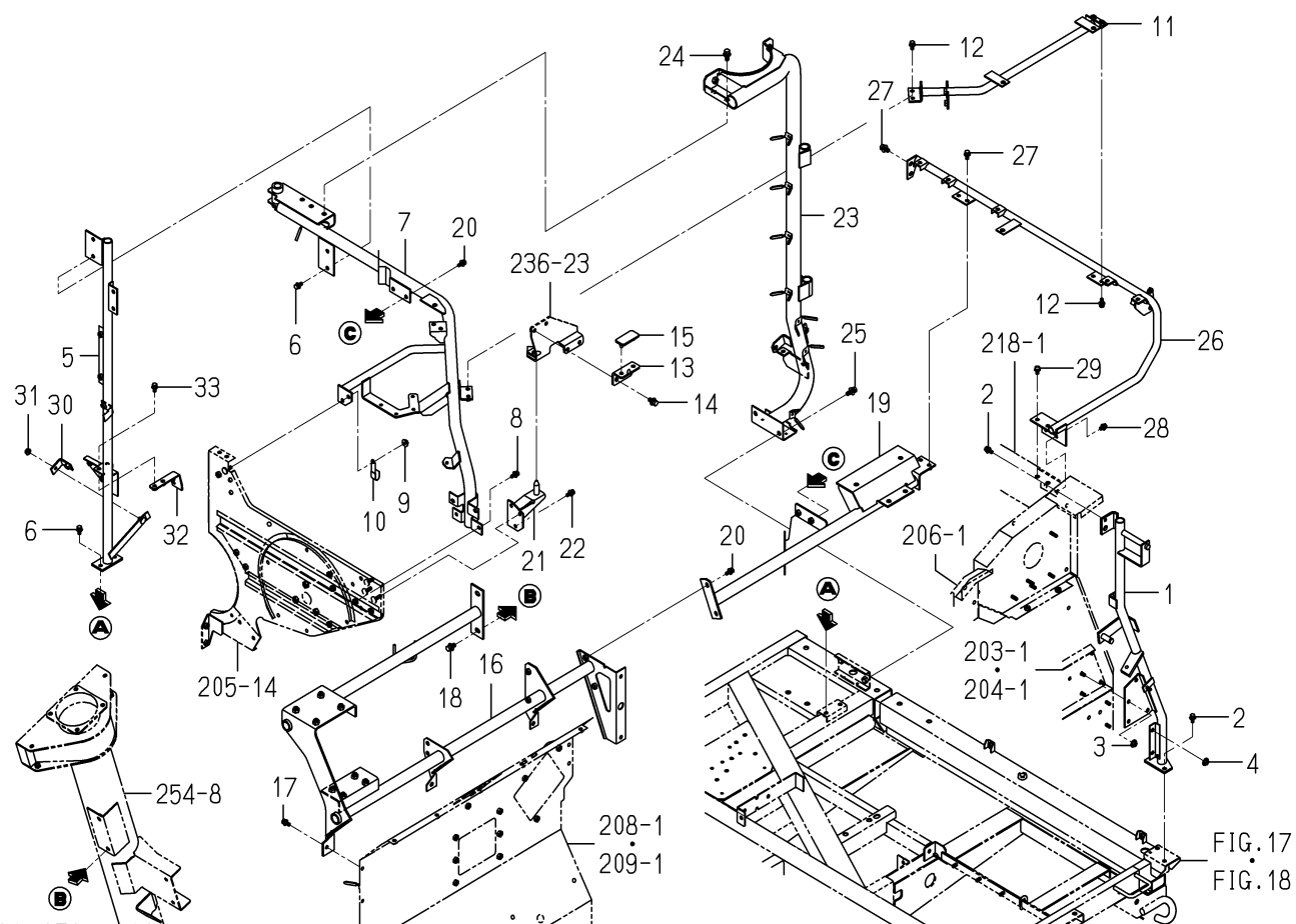
FIG.221 フレーム(リヤ)関係
