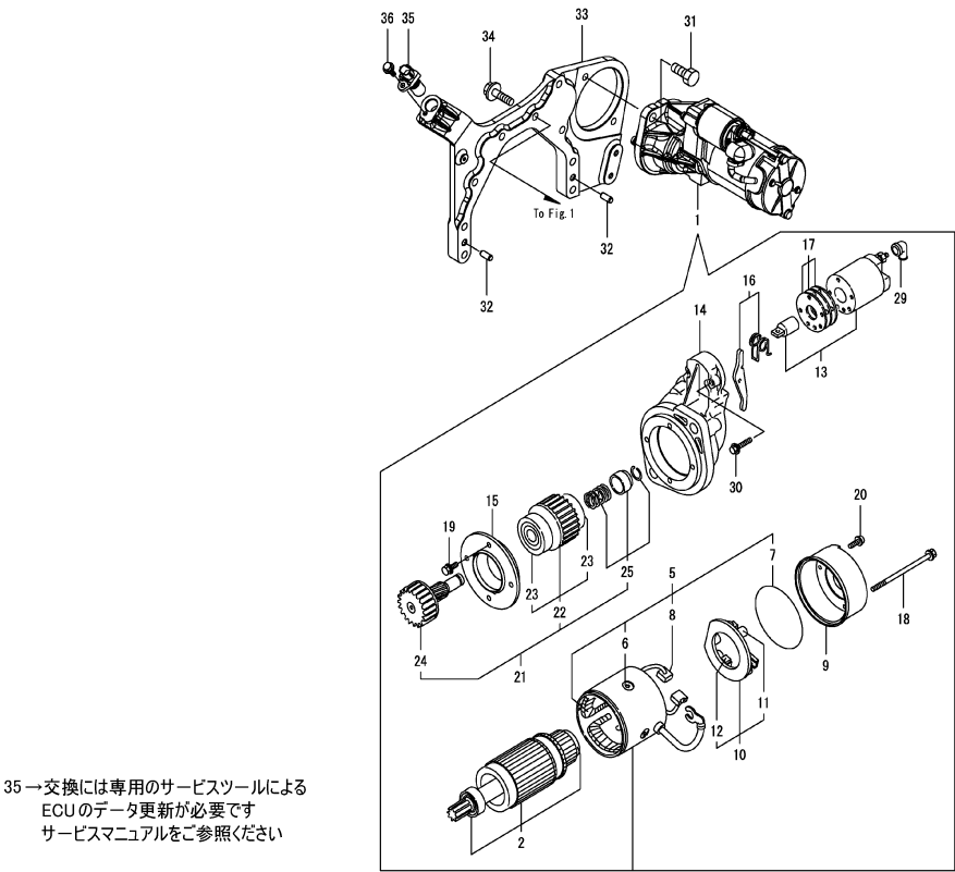
FIG.017 スタータモータ
