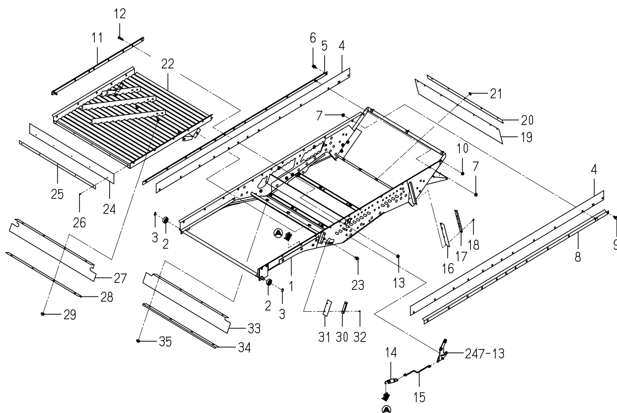
FIG.246 セパレータ関係
