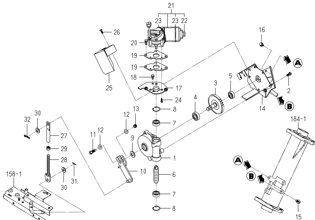
FIG.161 モータ(コギフカサ)関係
