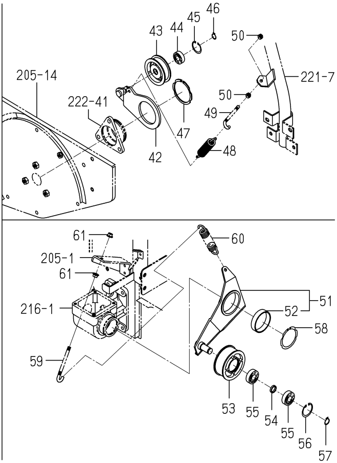
FIG.225 テンション(ベルト)関係(図2/2)
