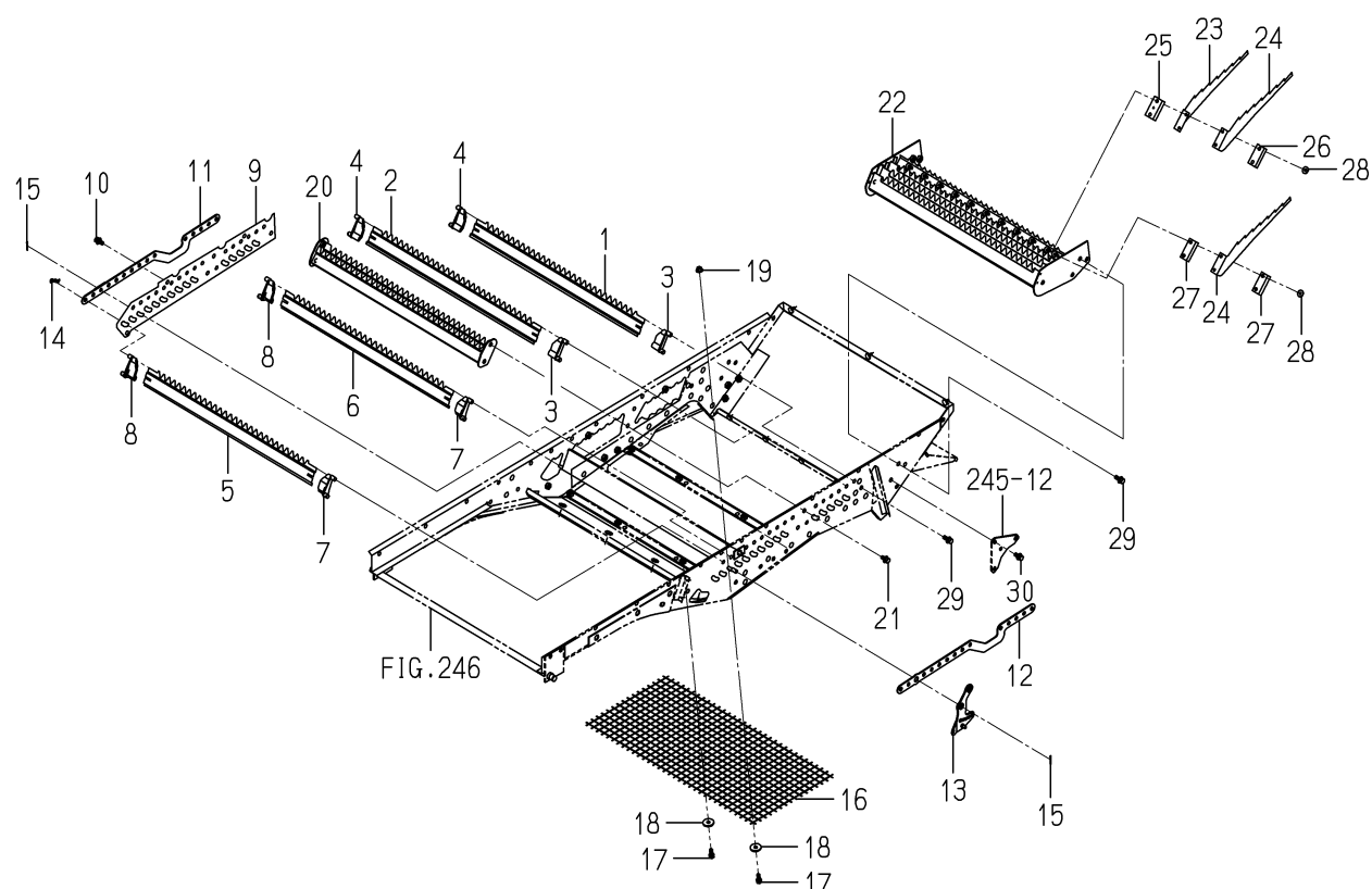
FIG.247 シーブ関係(図1/2)
