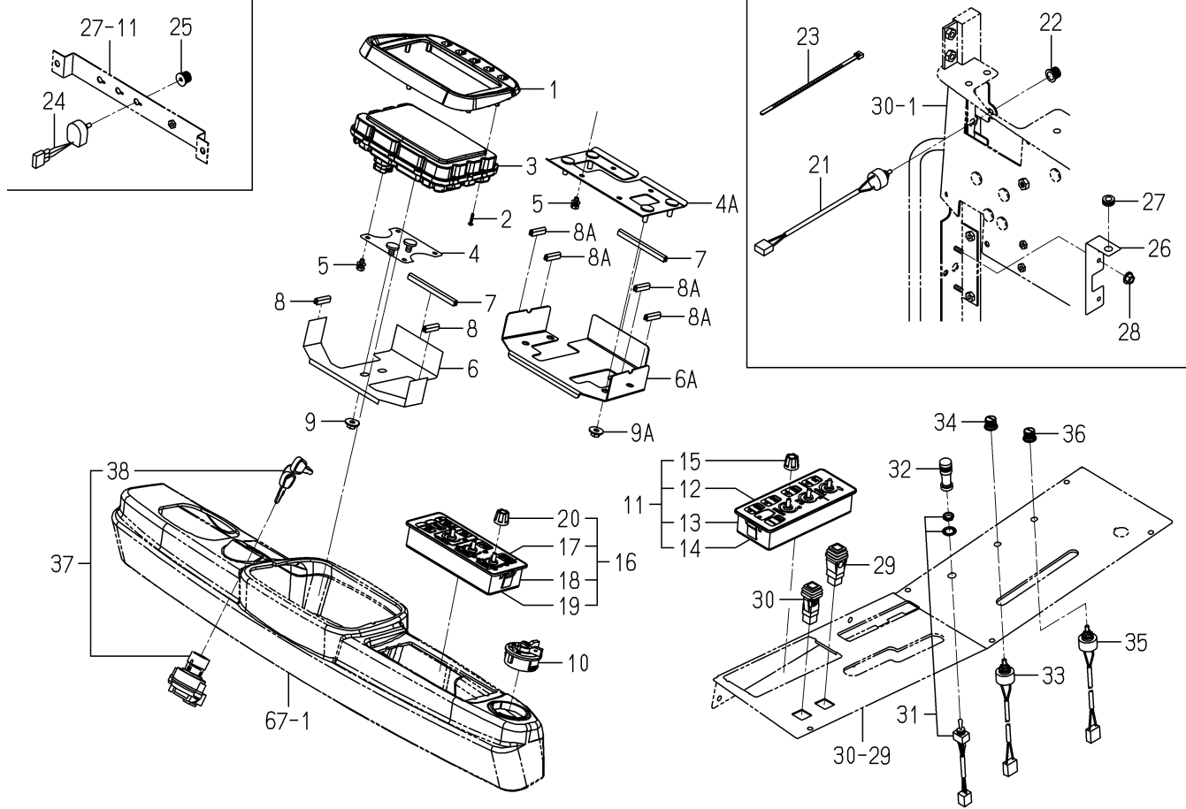
FIG. 65 パネル(インストルメント)関係(ZC型除く)
