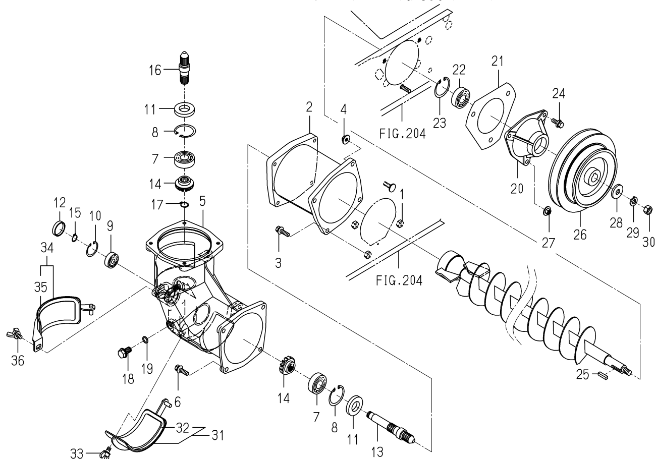
FIG.249 スパイラル(1ST)関係(T型)
