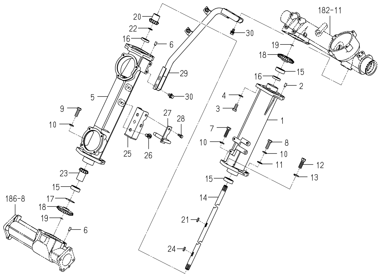
FIG.184 ケース(ギヤー／リヤ)関係
