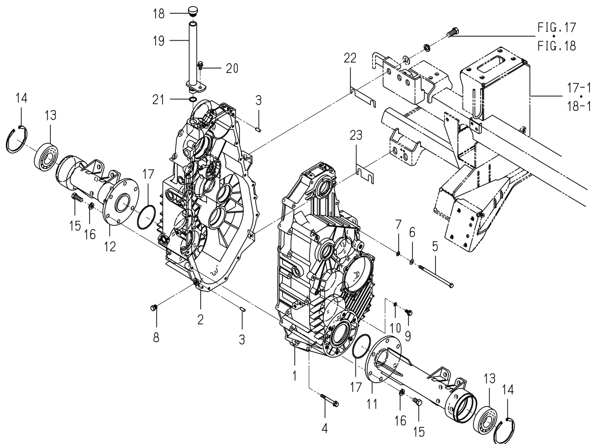
FIG. 1 ケース(トランスミツション)関係
