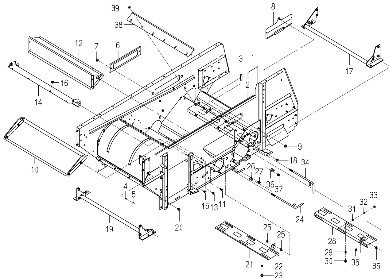
FIG.204 ホンタイ(1)関係(T型)(図1/2)
