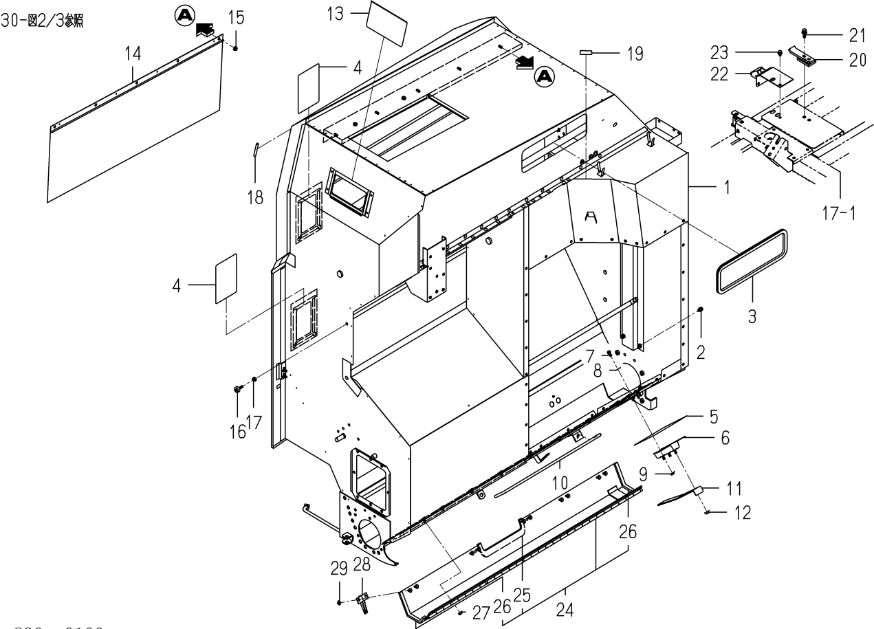
FIG.255 タンク(グレン)関係(A型)(図1/3)
