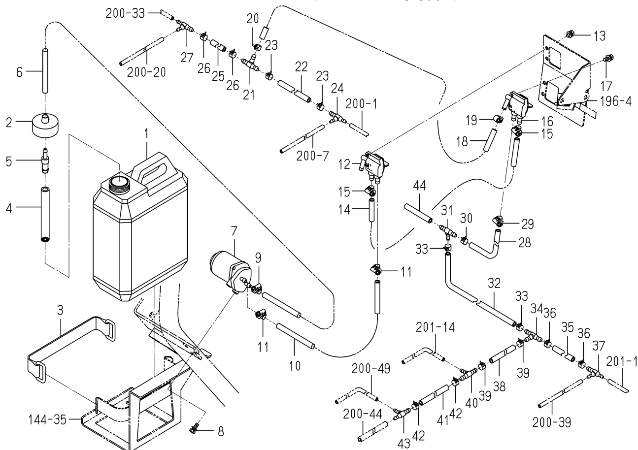
FIG.199 パイピング(オイリング)関係(図1/2)
