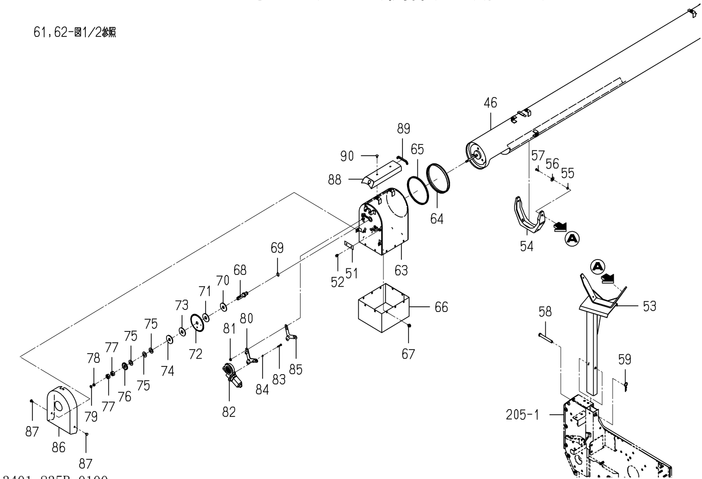
FIG.261 オーガ(アツパ)関係(T型)(図2/2)
