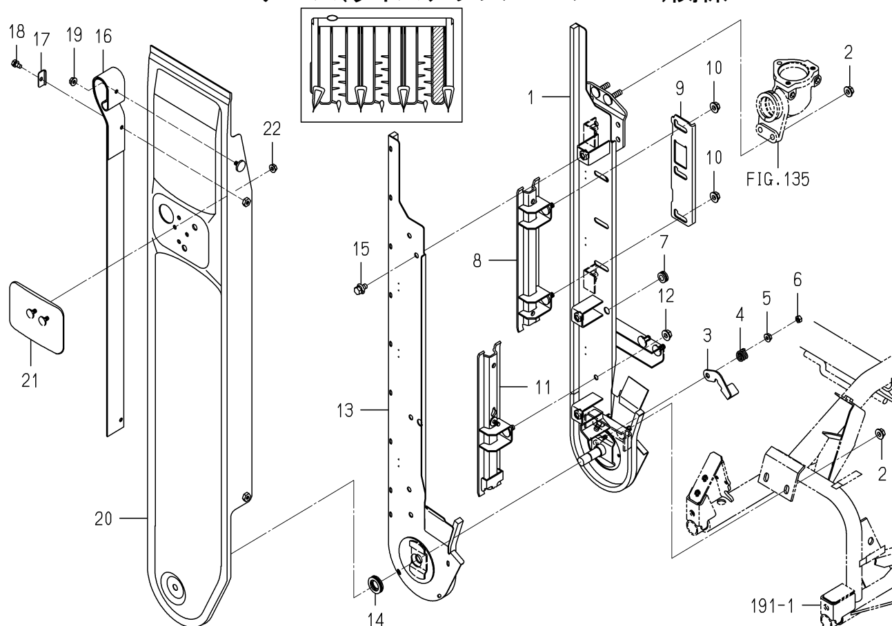
FIG.124 ケース(ライズアップ/LH/1ST)関係
