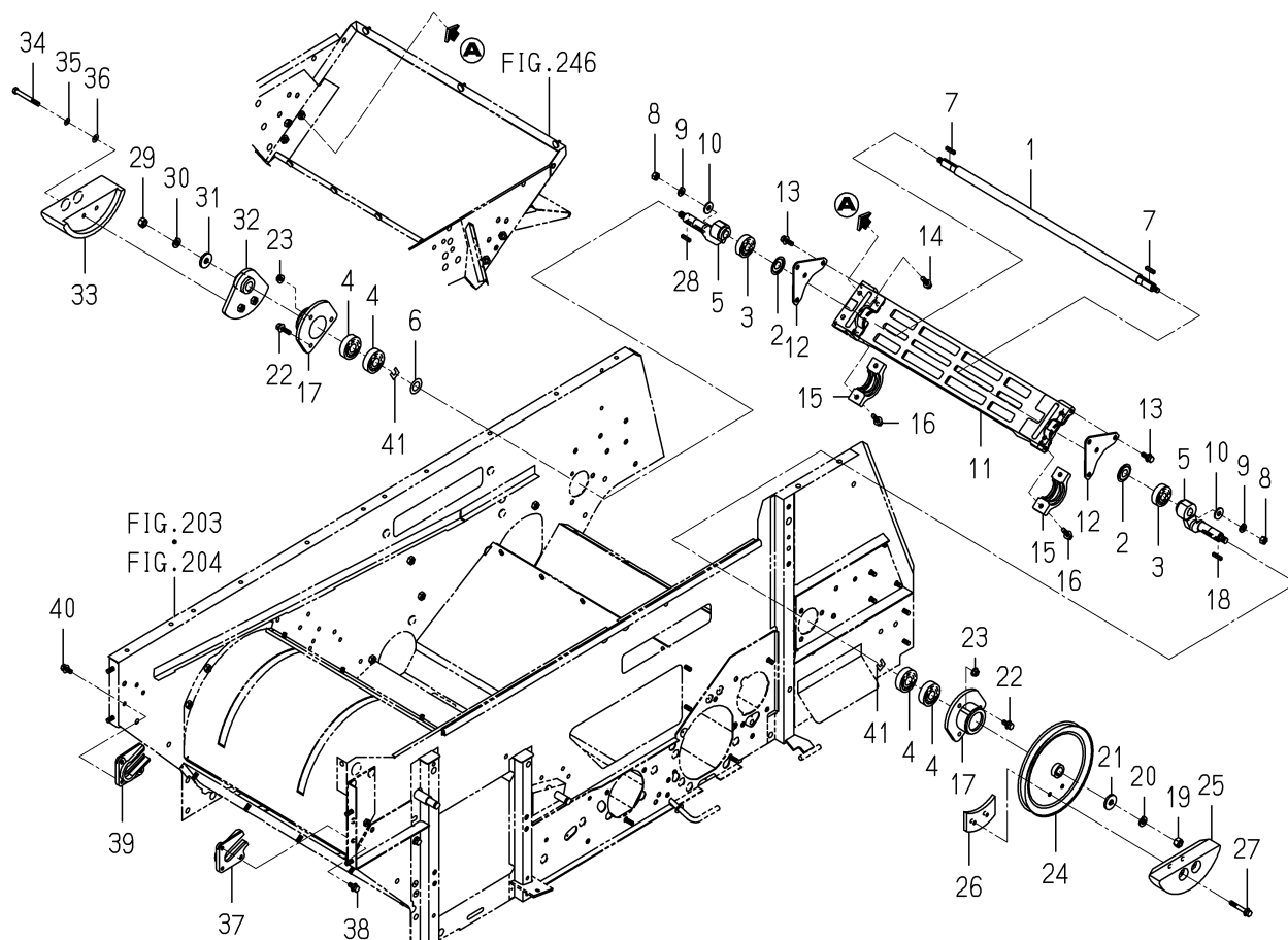
FIG.245 ドライブ(セパレータ)関係
