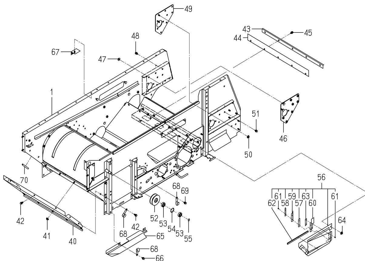
FIG.203 ホンタイ(1)関係(Z型)(図2/2)
