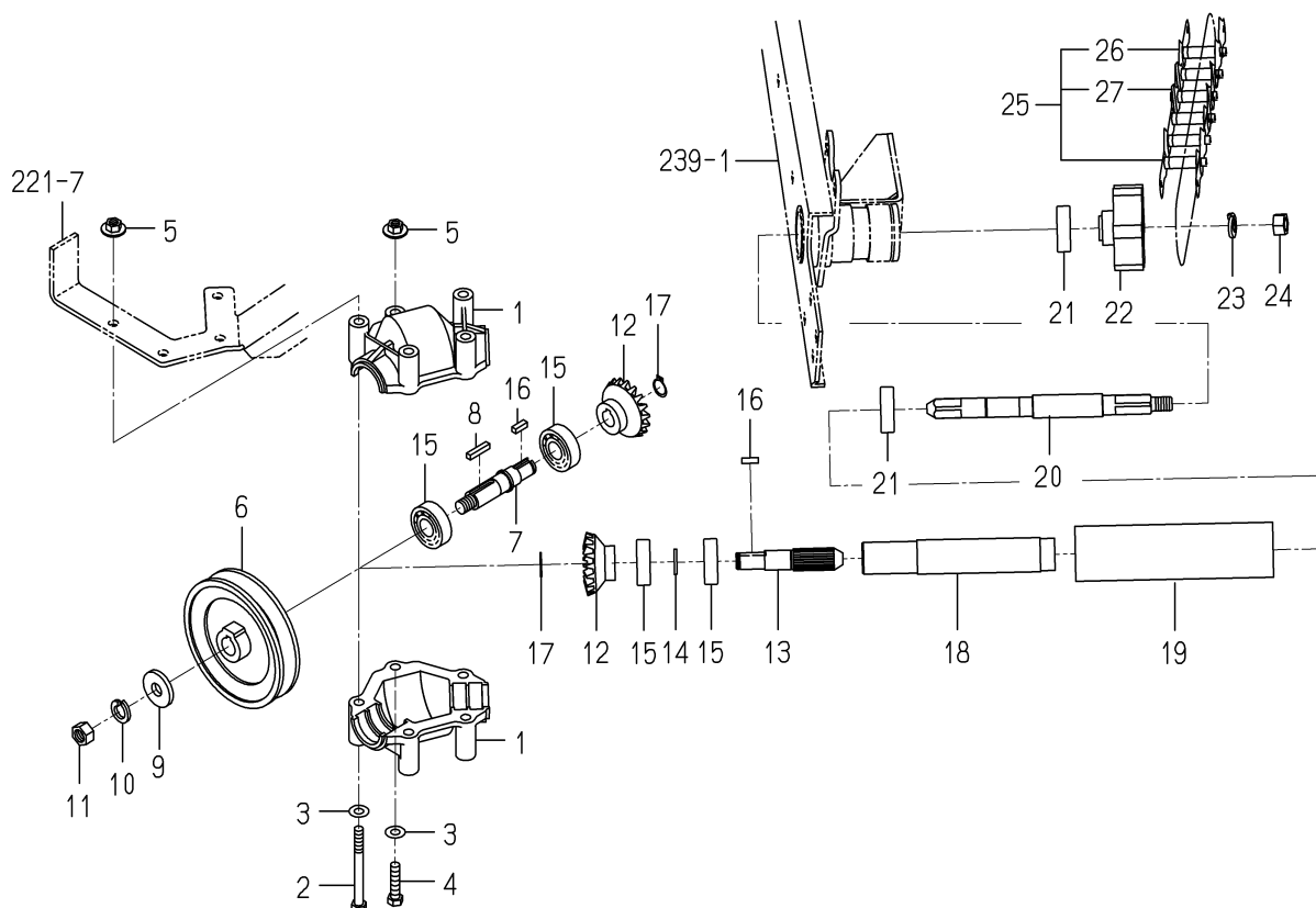
FIG.235 インพุット(エジエクタ／ストーク)関係(T型)
