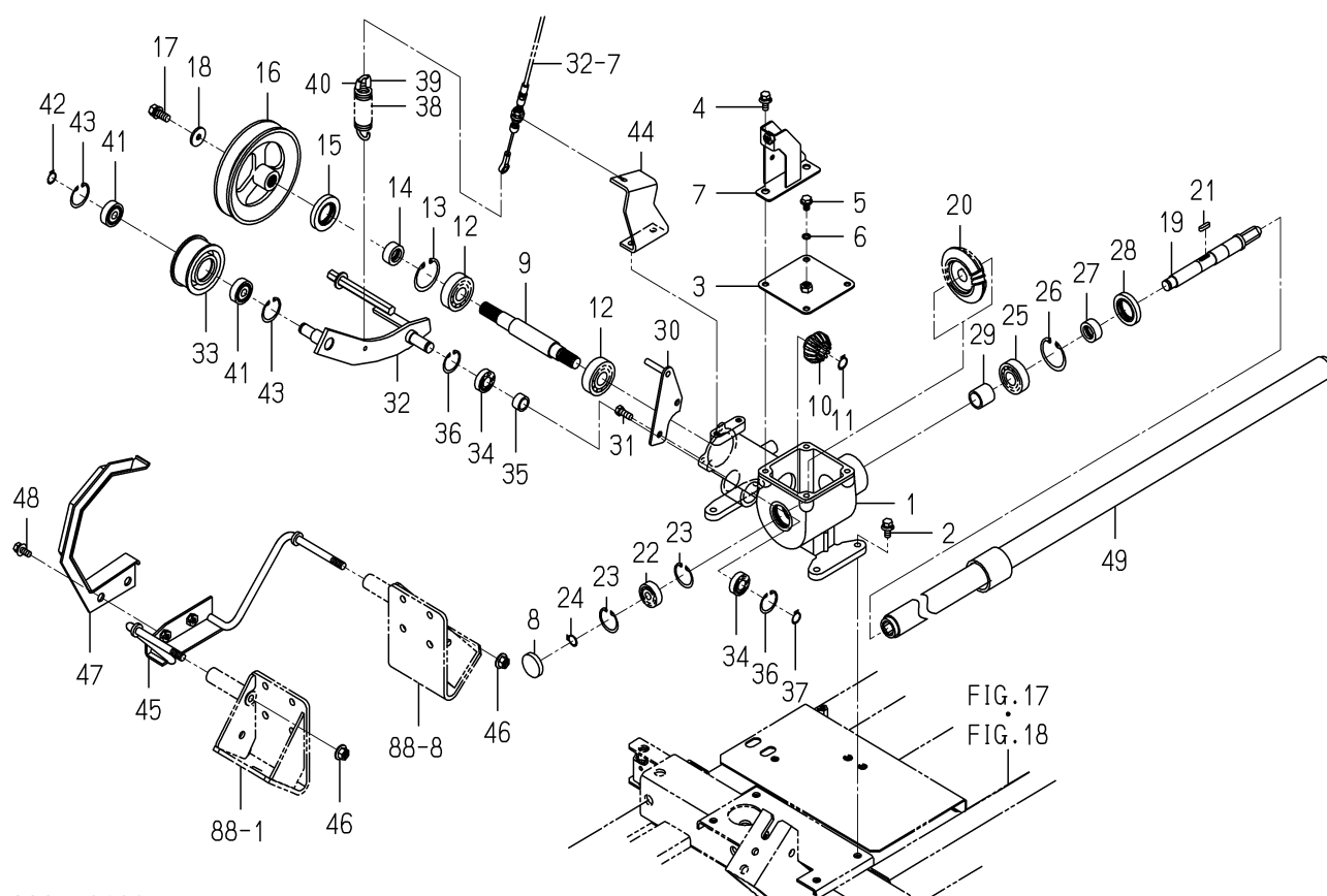
FIG.257 ドライブ(タンク/グレン)関係(図1/2)
