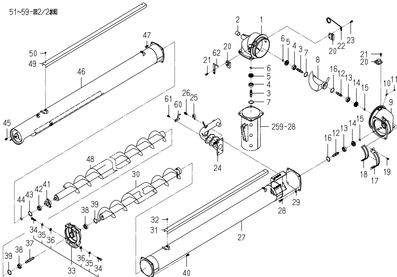
FIG.261 オーガ(アツパ)関係(T型)(図1/2)
