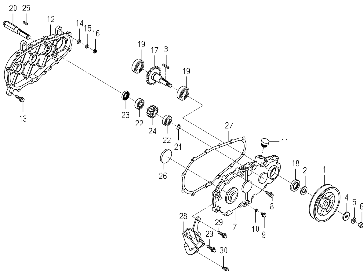
FIG.223 ドライブ(エジェクタ)関係(Z型)
