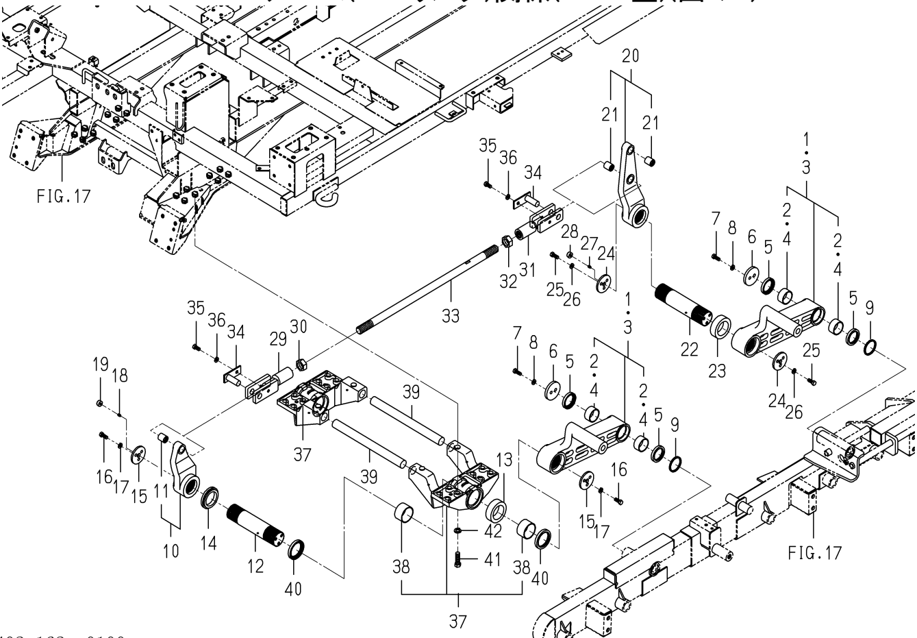
FIG. 20 アーム(ローリング)関係(LHW型)(図1/2)
