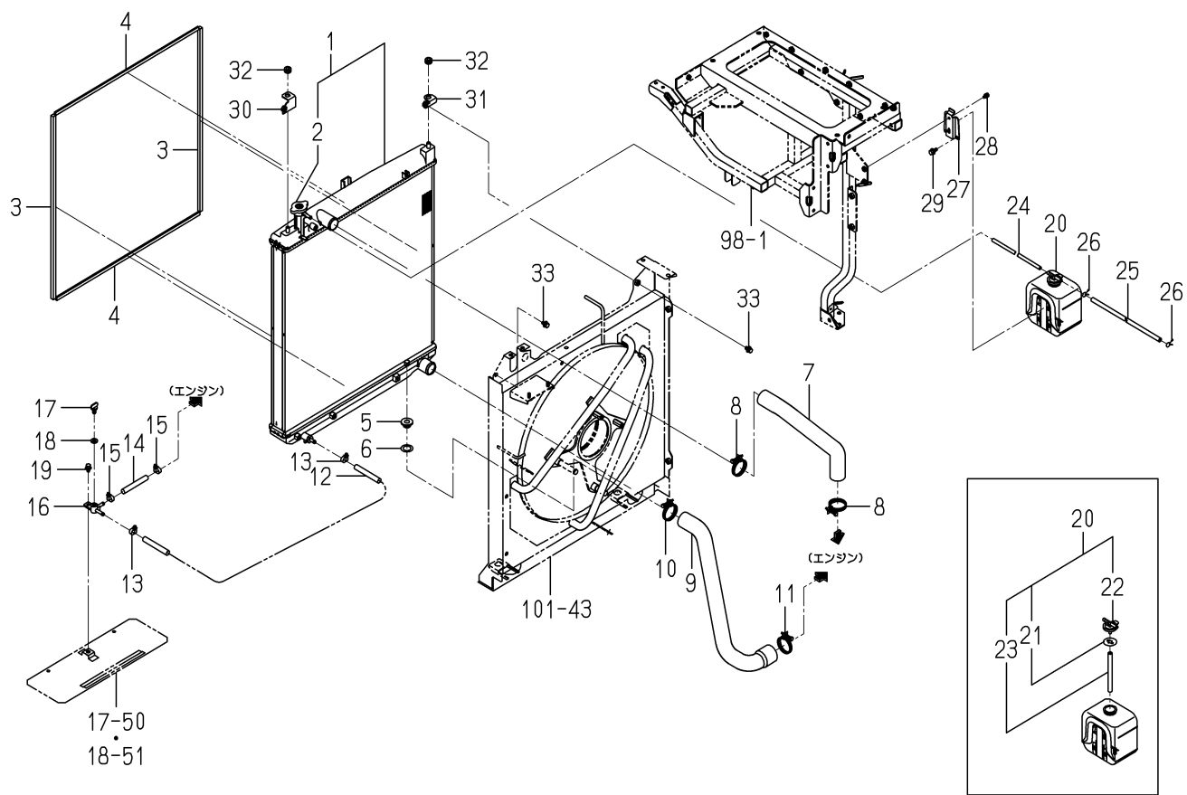
FIG. 93 ラジエータ関係(ZC型)(図1/2)
