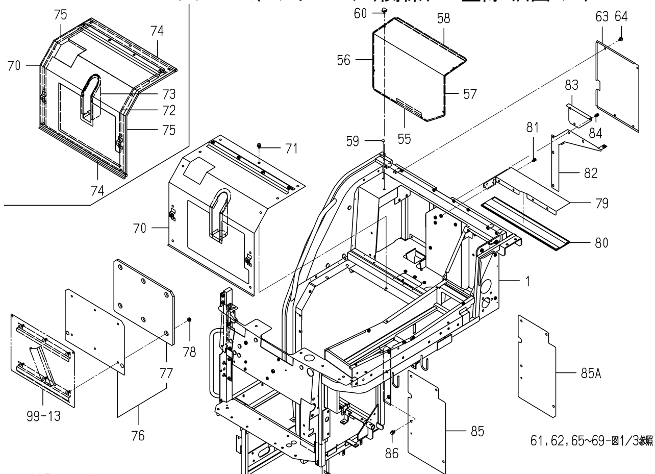
FIG. 30 フレーム(コントロール)関係(ZC型除く)(図3/3)
