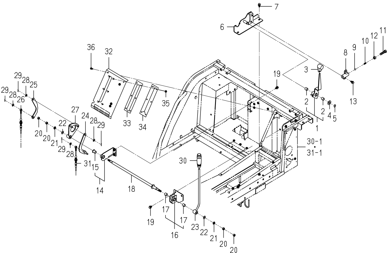
FIG. 39 レバー(カリトリ, ダツコク)関係
