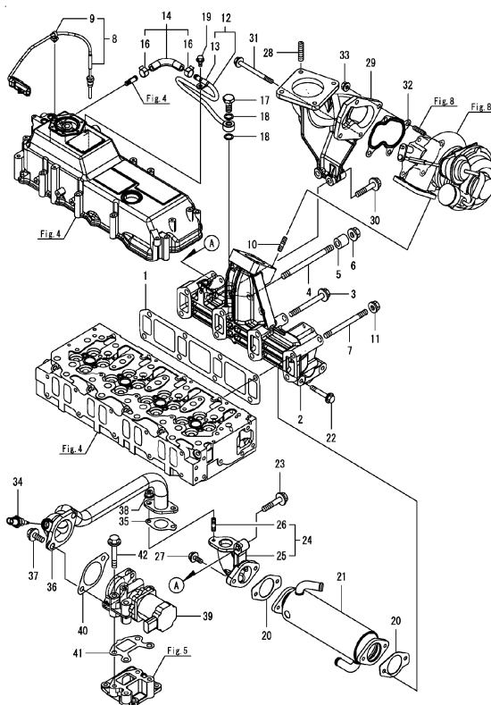
FIG.006 排気マニホールド
