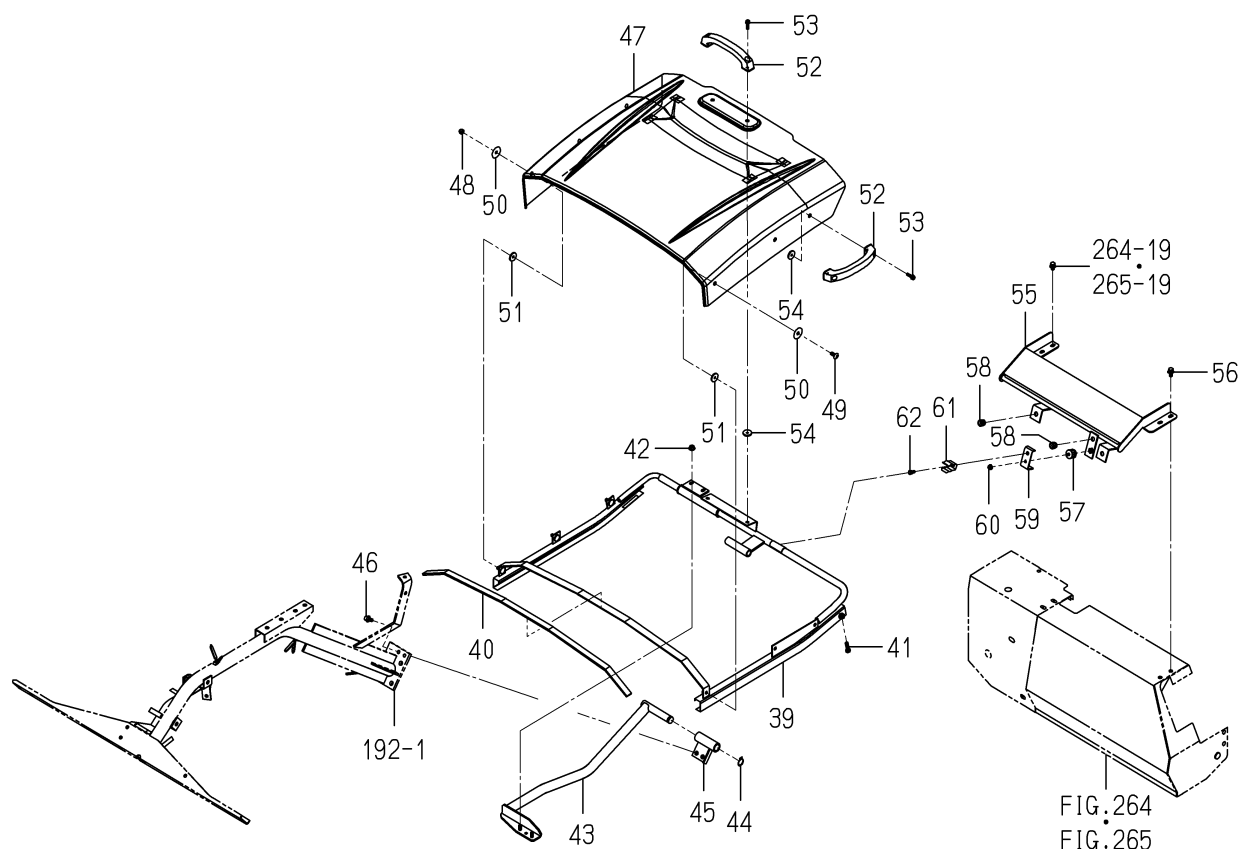
FIG.197 カバー(ダスト)関係(ZC型除く)(図2/2)
