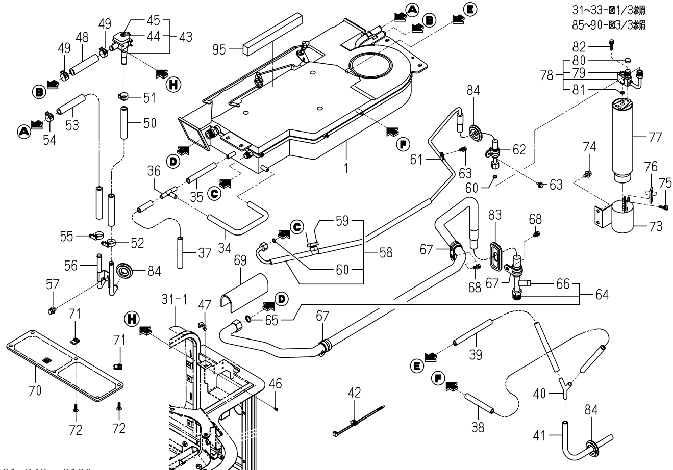
FIG. 53 エアコン(キャビン)関係(ZC型)(図2/3)
