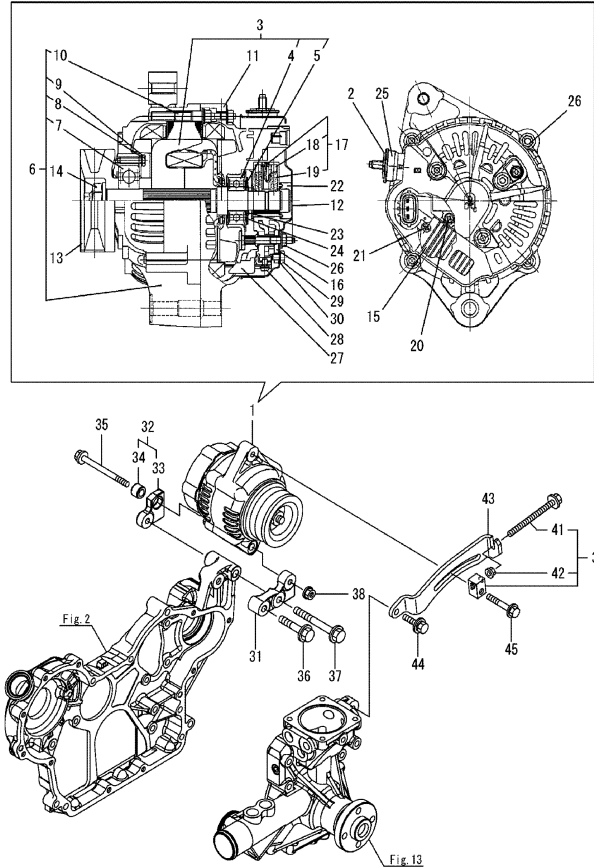
FIG.018 ジェネレータ
