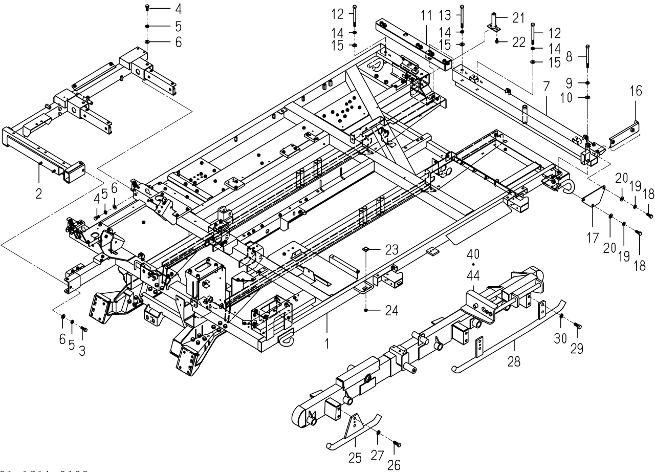
FIG. 18 フレーム(ソウコウ／オープン)関係(S型)(図1/2)
