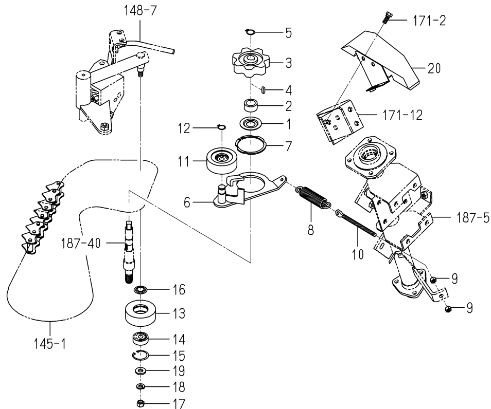
FIG.146 ドライブ(ネモト／LH)関係
