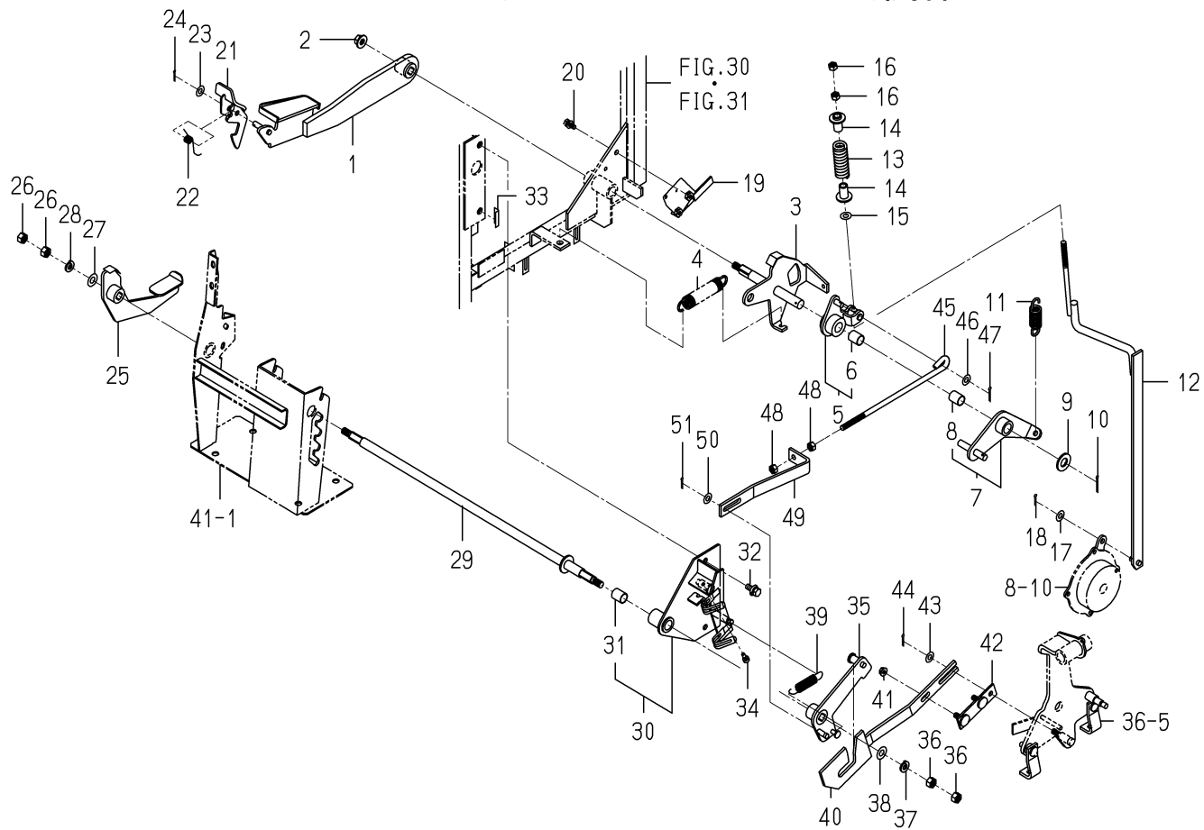
FIG. 42 ペダル(ブレーキ／パーキング)関係
