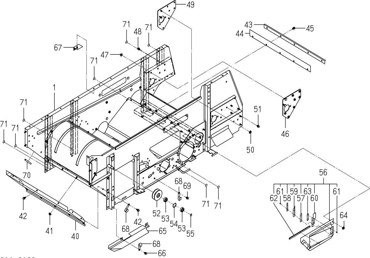
FIG.204 ホンタイ(1)関係(T型)(図2/2)
