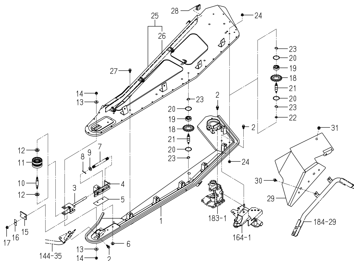
FIG.178 ケース(ホサキ/センタ)関係
