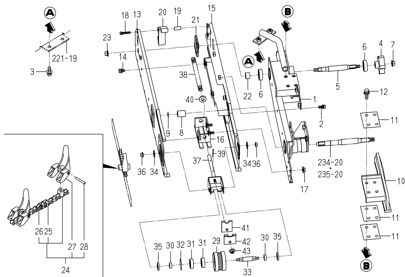
FIG.239 レール(エジクタ/ストーク/ホサキ)関係
