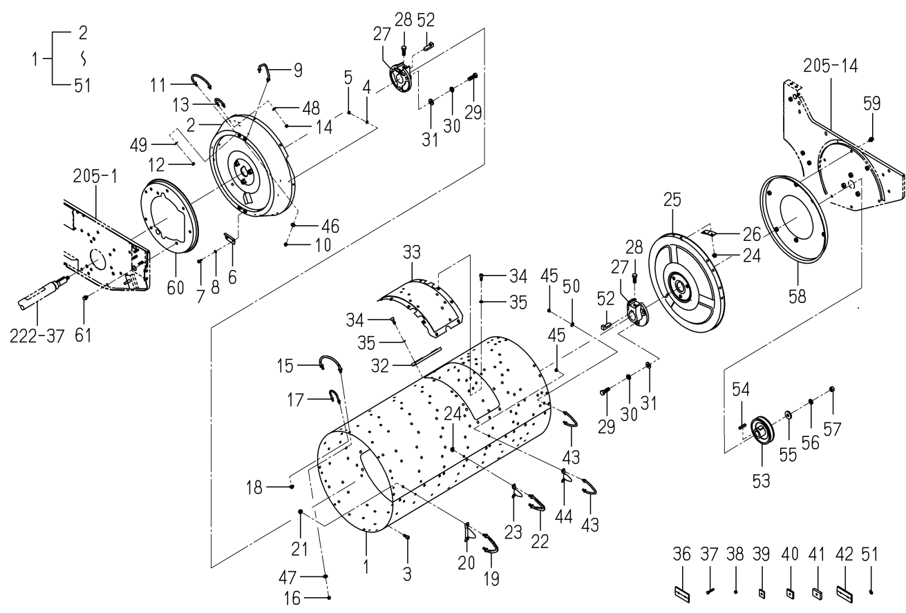
FIG.210 シリンダ関係
