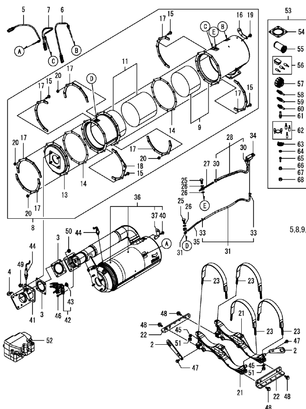
FIG.024 ATDユニット
