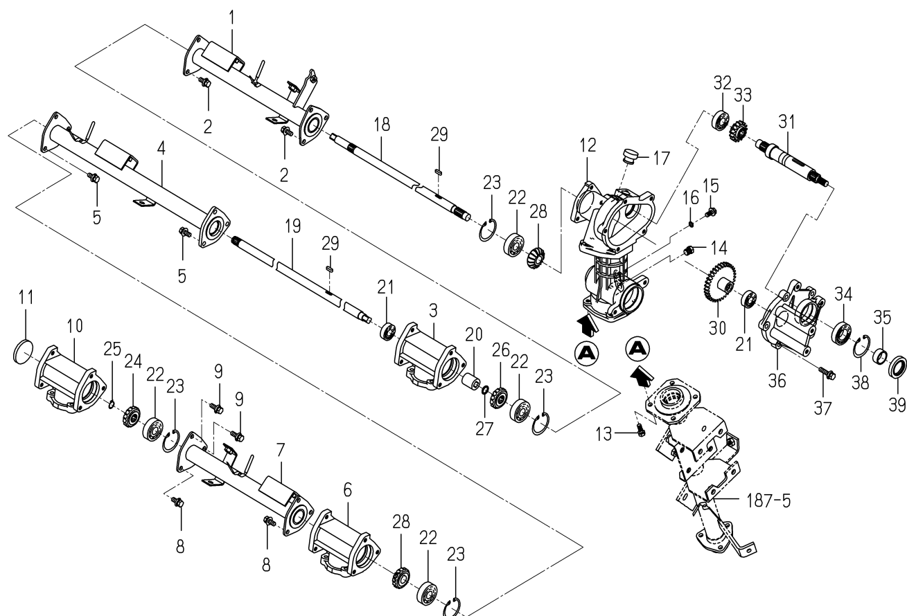
FIG.188 ケース(ギヤー／アツパ)関係
