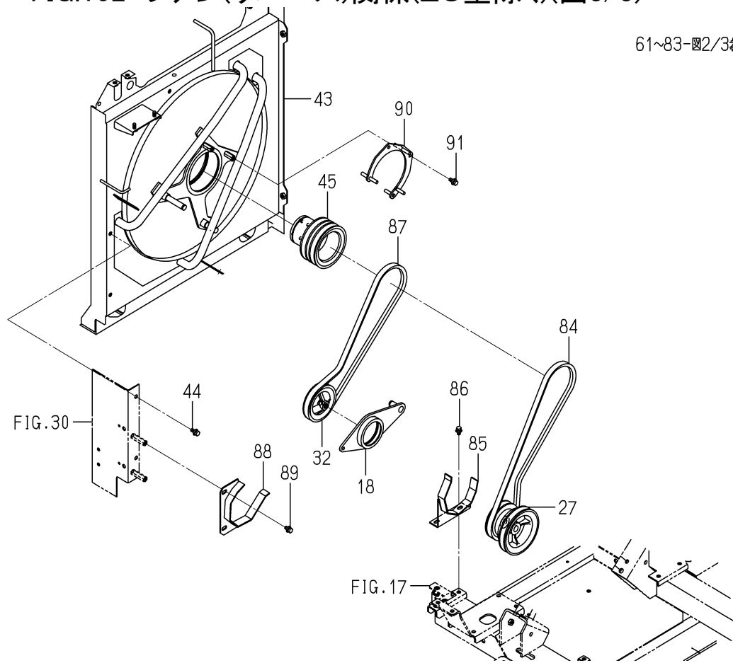
FIG.102 ファン(リバーズ)関係(ZC型除く)(図3/3)
