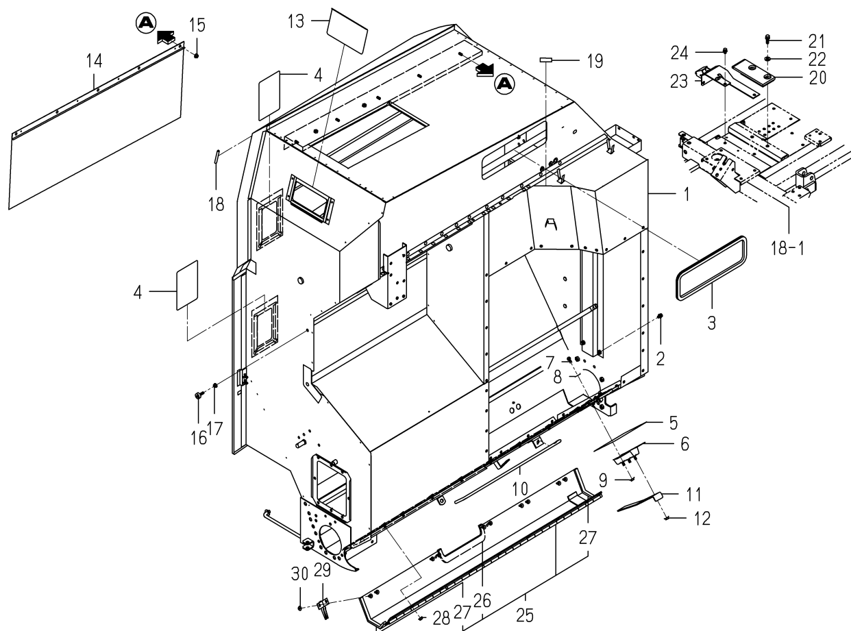
FIG.256 タンク(グレン)関係(S型)(図1/4)
