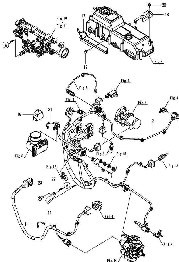
FIG.023 電装品
