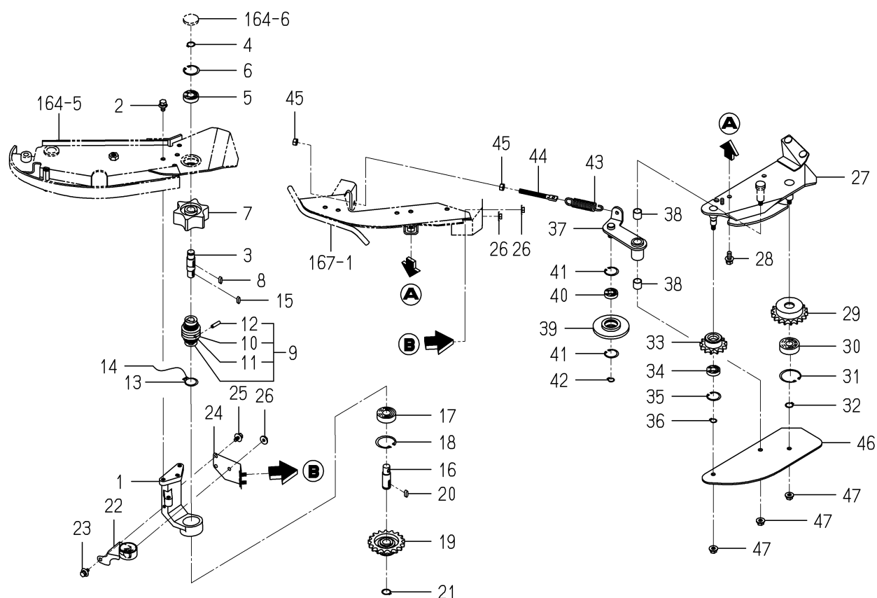
FIG.169 フレーム(キョウキュウ/ロー)関係
