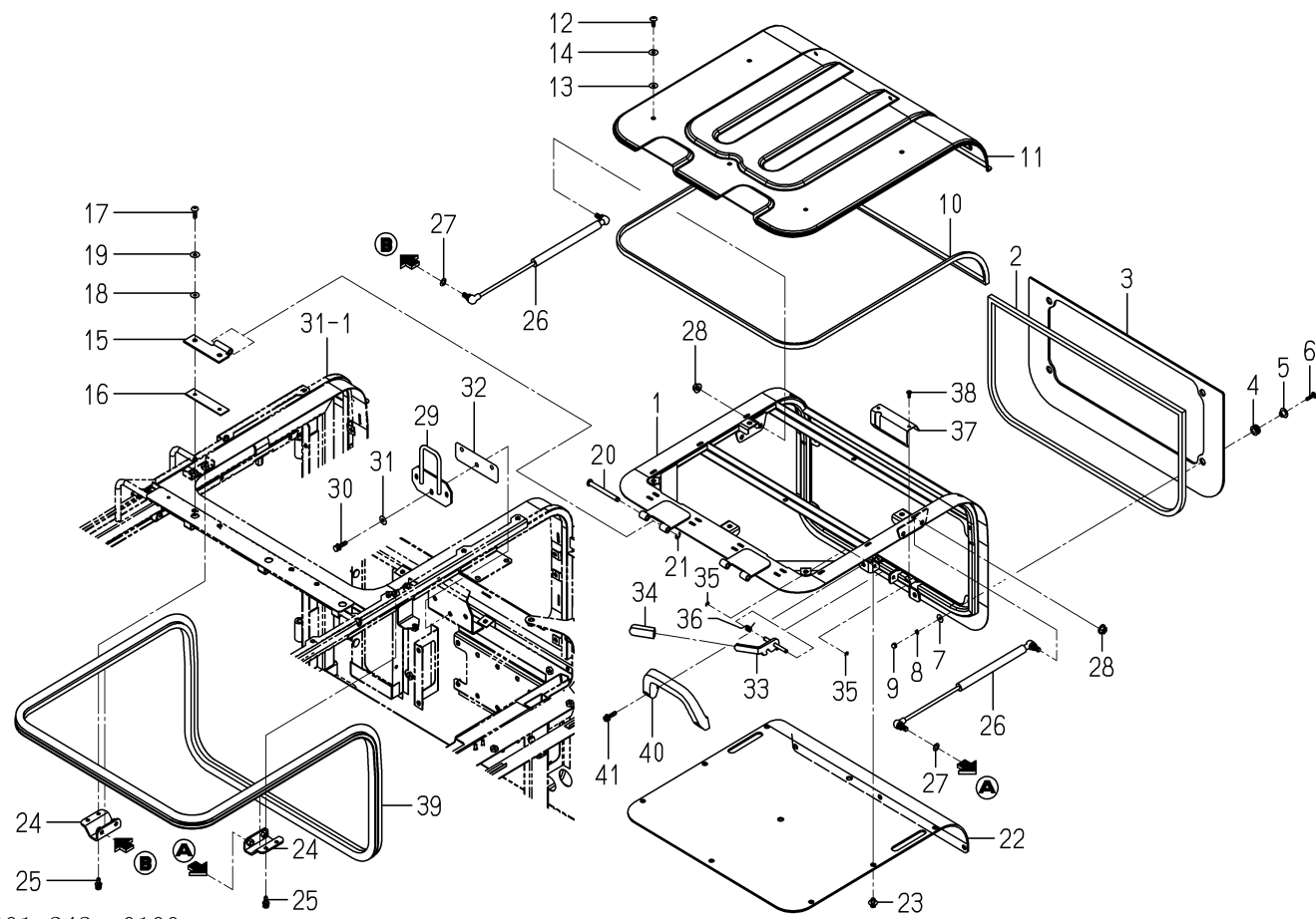
FIG. 50 ハッチ(リヤ／キャビン)関係(ZC型)
