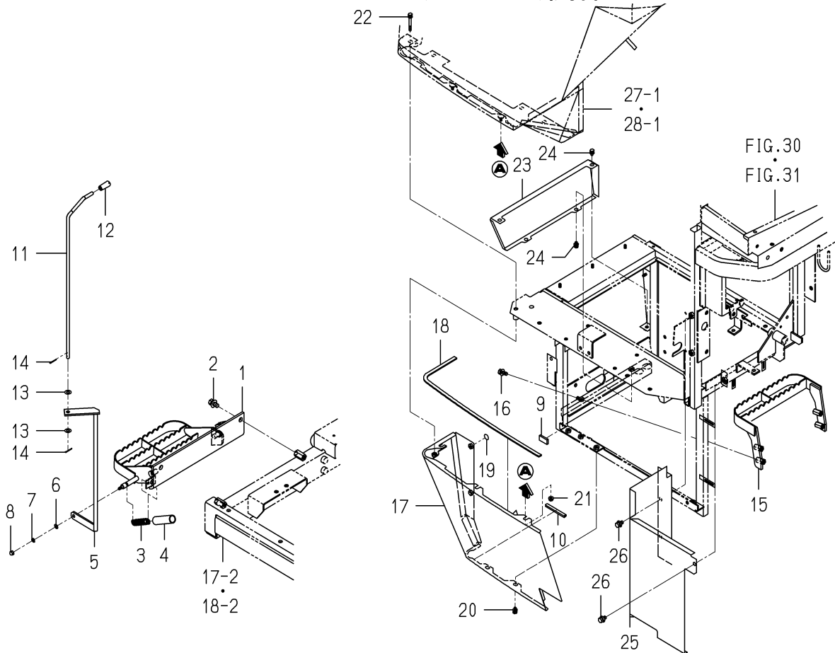
FIG. 29 カバー(フレーム)関係
