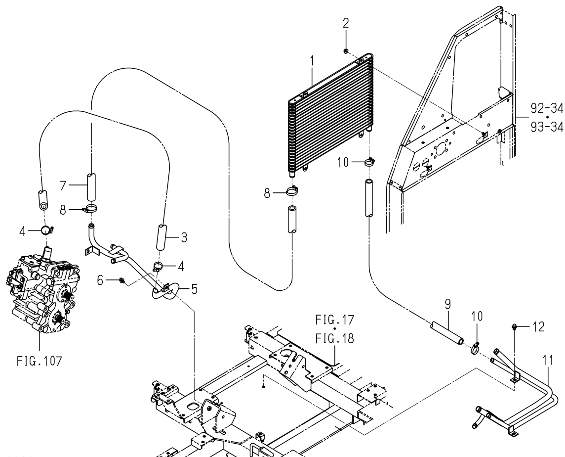
FIG.110 クーラ(オイル)関係
