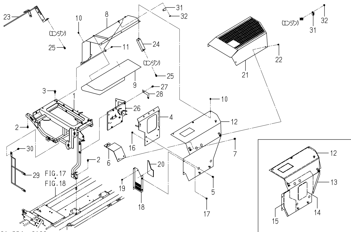
FIG. 98 カバー(エキゾースト)関係
