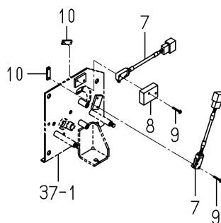
FIG. 77 センサ(ソウコウ)関係(図1/2)
