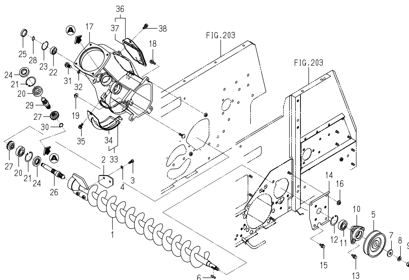
FIG.250 スパイラル(2ND)関係(Z型)
