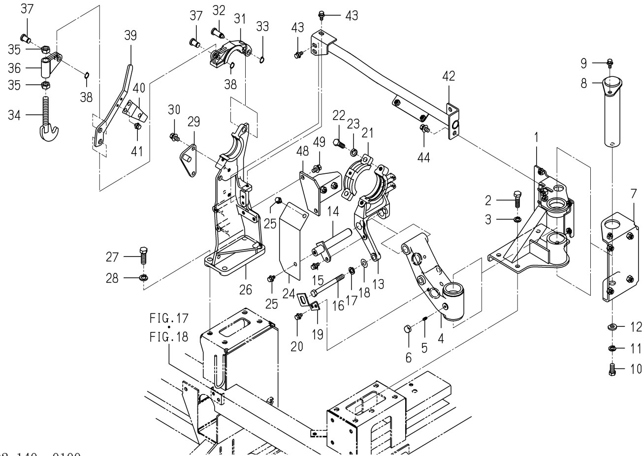
FIG. 14 ベース(オープン／カトリ)関係(図1/2)
