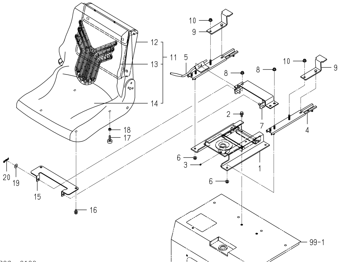
FIG. 32 シート関係
