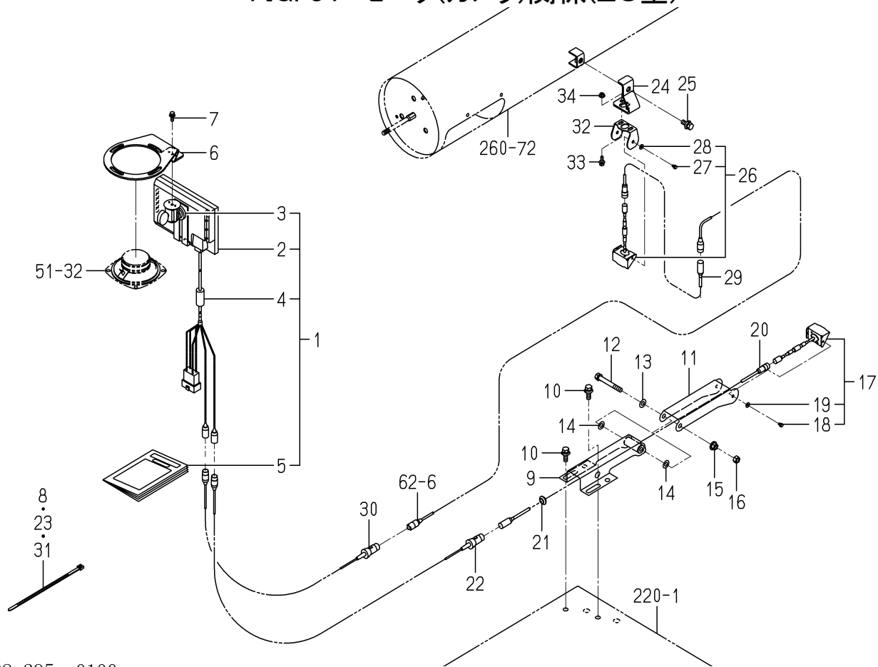
FIG. 84 モニタ(カメラ)関係(ZC型)
