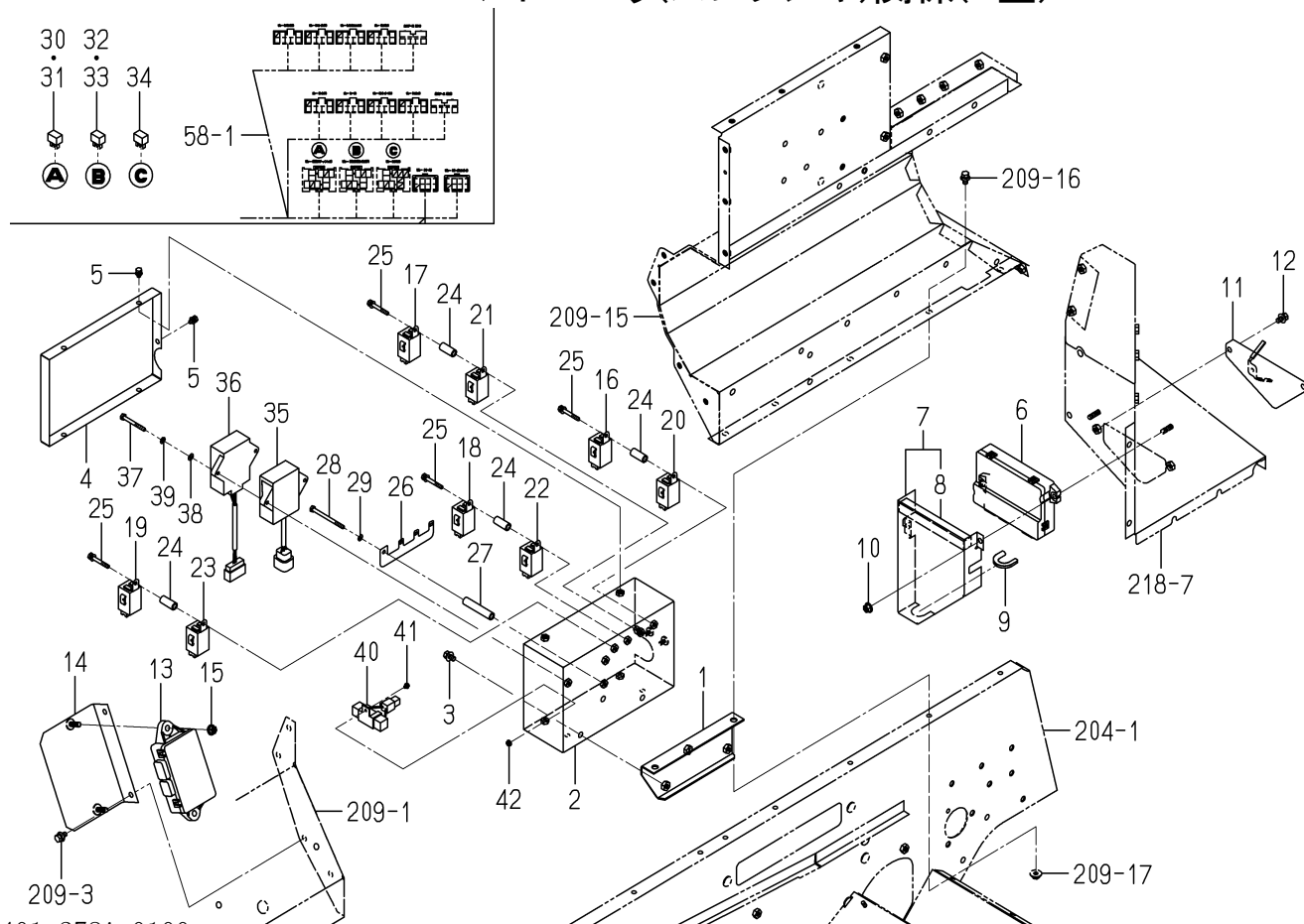
FIG. 74 コントローラ(スレッシヤ)関係(T型)
