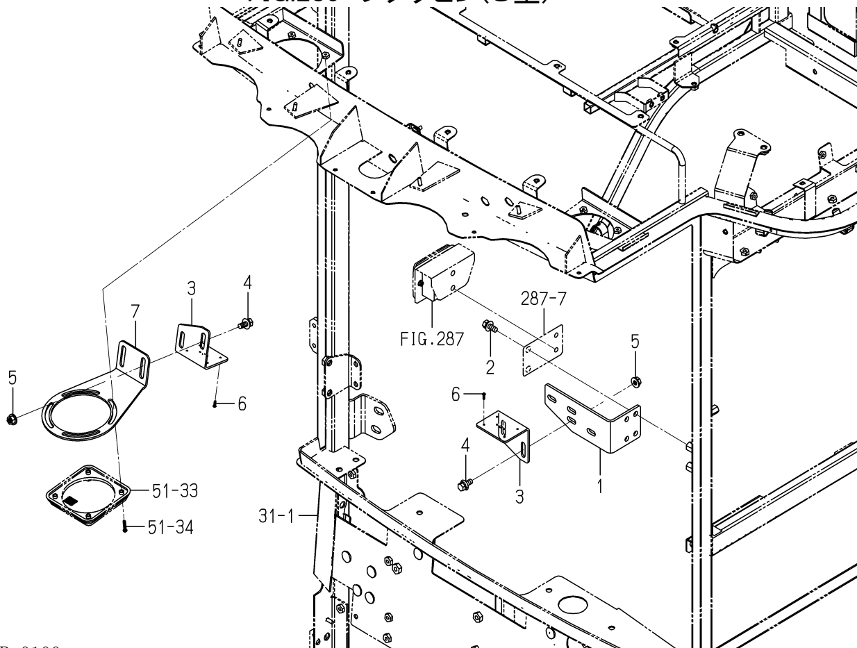
FIG.285 フゾクヒン(S型)
