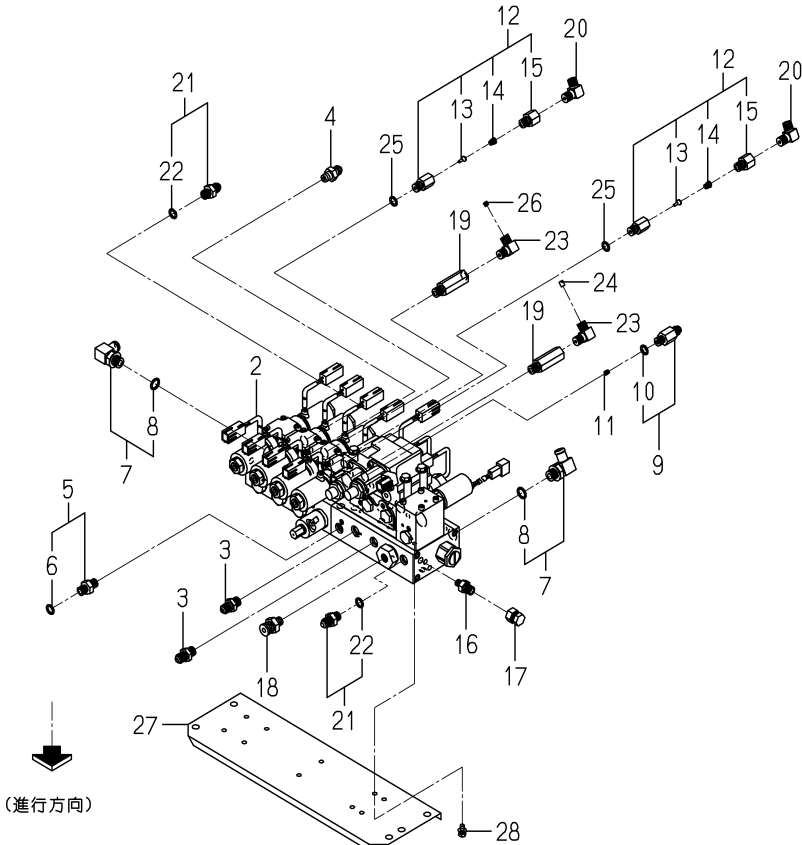
FIG.105 バルブ(図1/2) (コントロール／ローリング&ピッチング)関係
