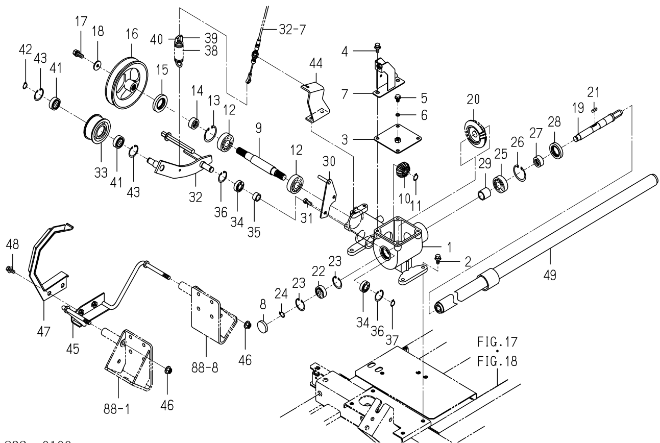
FIG.257 ドライブ(タンク/グレン)関係(図1/2)
