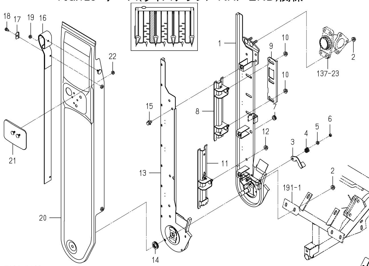
FIG.128 ケース(ライズアップ/RH/2ND)関係
