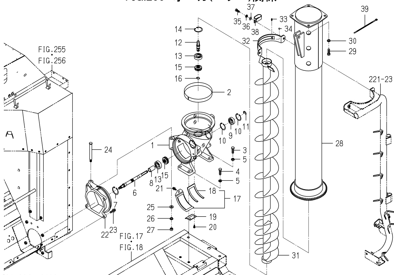
FIG.259 オーガ(ロー)関係
