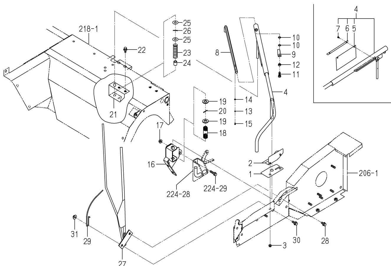
FIG.238 ホルダ(エジェクタ/ストーク)関係(T型)
