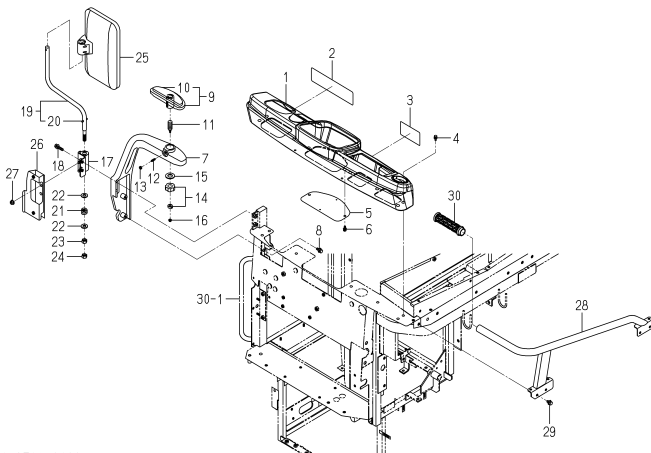
FIG. 67 パネル(スイッチ/フロント)関係(ZC型除く)
