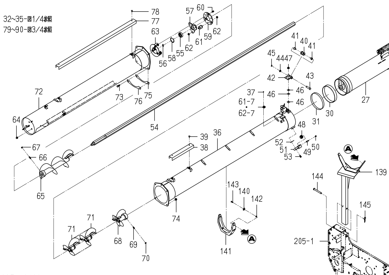
FIG.260 ドライブ(オーガ／スイング)関係(Z型)(図2/4)
