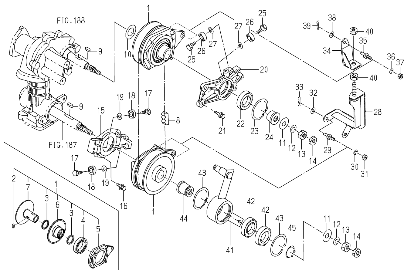
FIG.189 シンクロ関係(図1/2)
