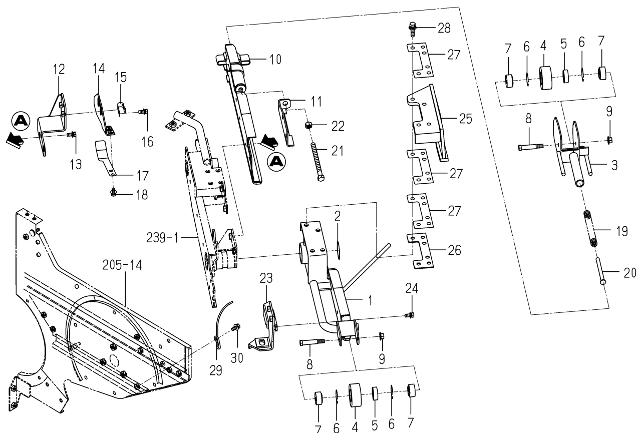
FIG.236 レール(エジクタ/ストーク/ネモト)関係
