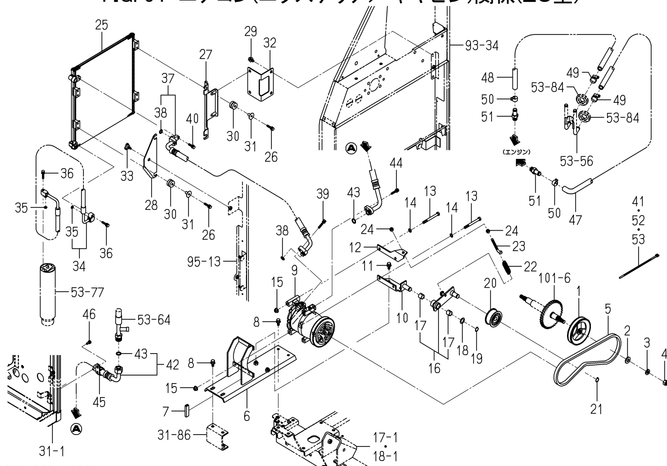
FIG. 54 エアコン(エクステリア/キャビン)関係(ZC型)
