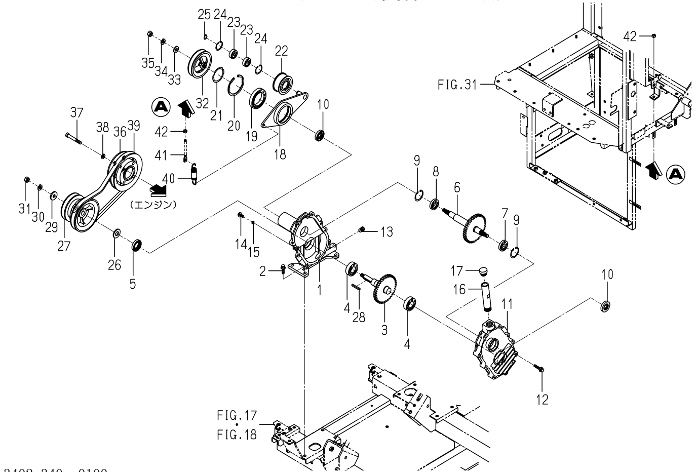
FIG.101 ファン(リバー)関係(ZC型)(図1/3)
