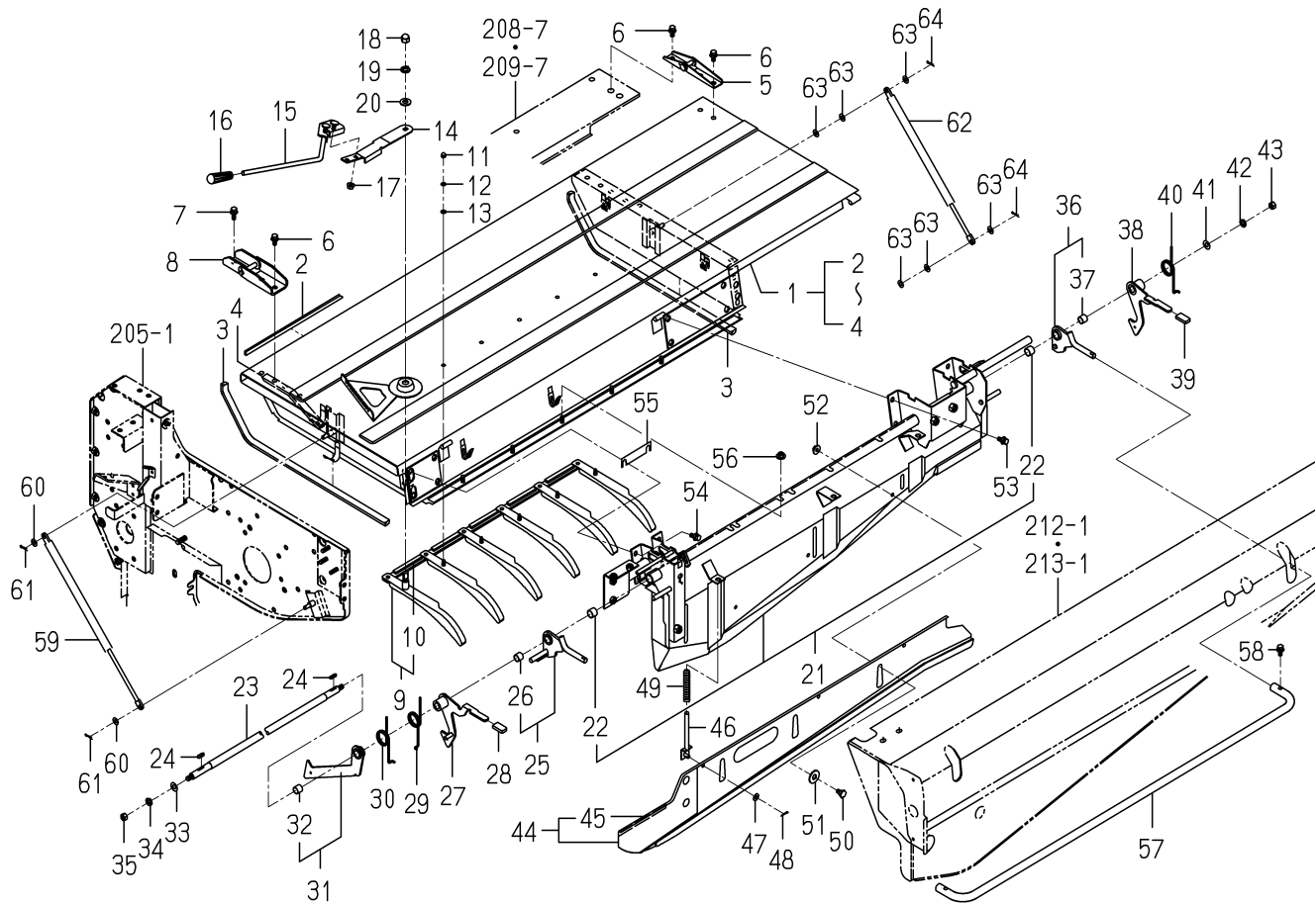
FIG.211 カバー(シリンダ)関係
