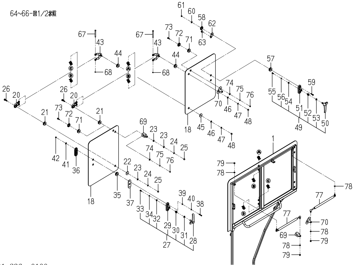
FIG. 47 ドア(キヤビン)関係(ZC型)(図2/2)
