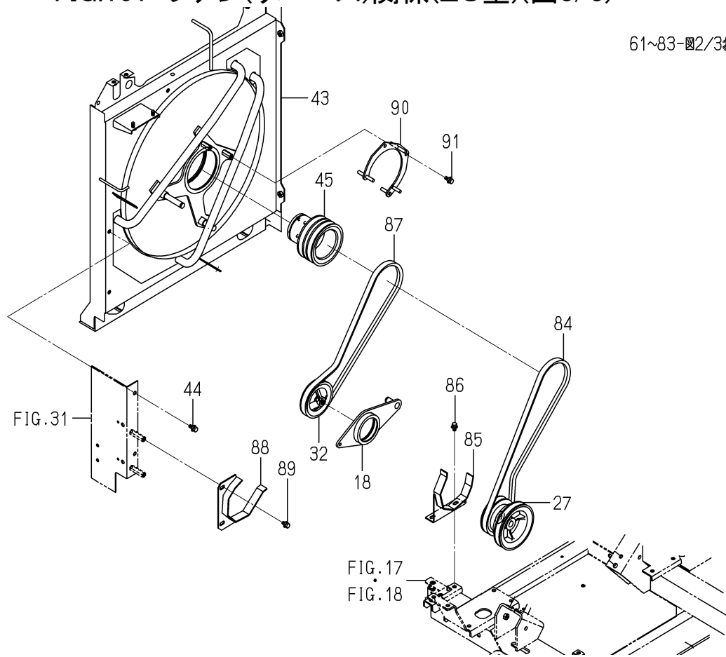
FIG.101 ファン(リバー)関係(ZC型)(図3/3)
