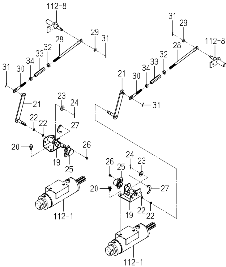
FIG. 77 センサ(ソウコウ)関係(図2/2)
