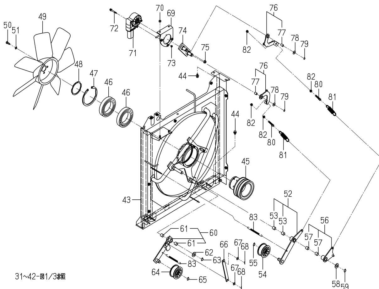
FIG.101 ファン(リバー)関係(ZC型)(図2/3)
