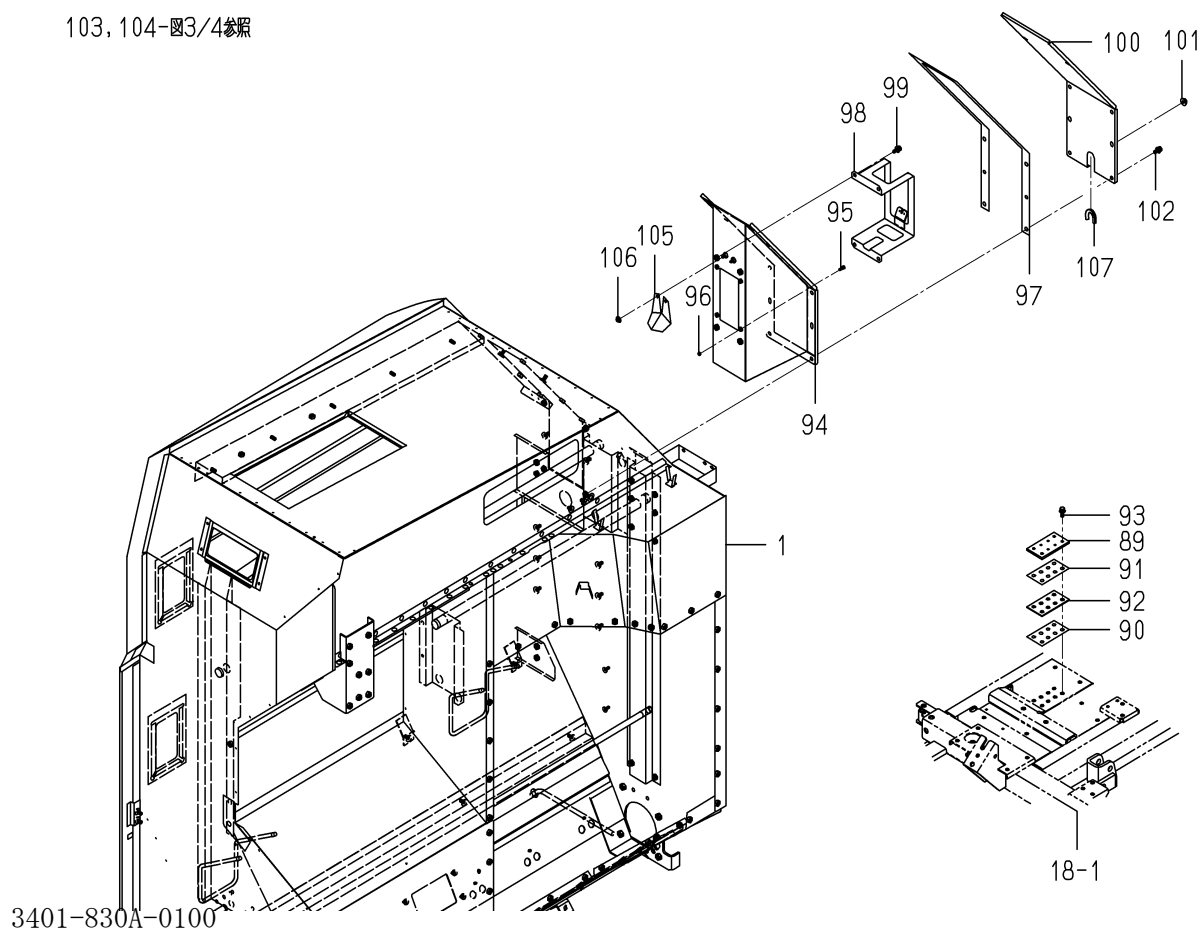
FIG.256 タンク(グレン)関係(S型)(図4/4)
