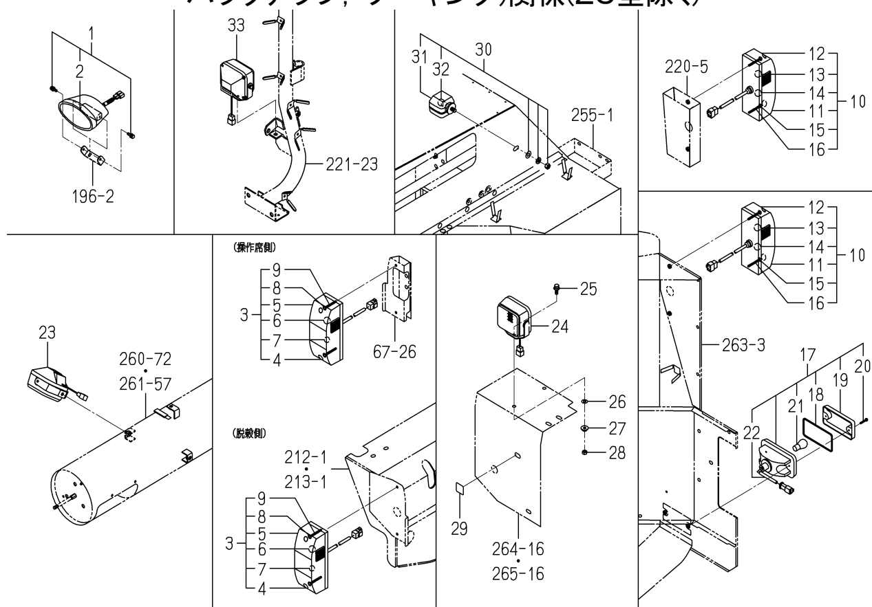
FIG. 82 ランプ(ヘッド, ターンシグナル, バックアップ, ワーキング)関係(ZC型除く)
