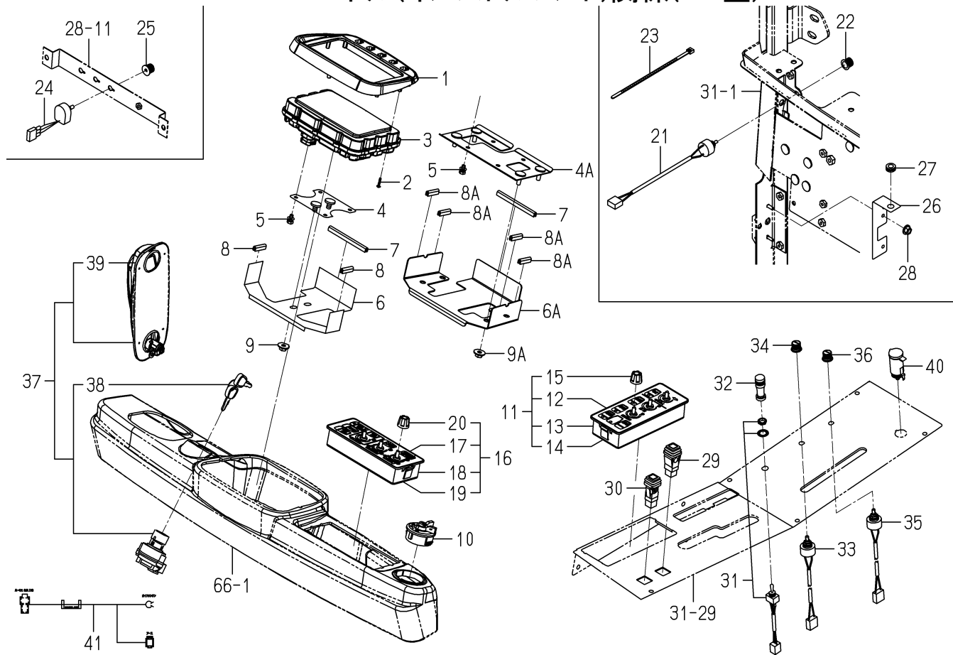
FIG. 64 パネル(インストルメント)関係(ZC型)
