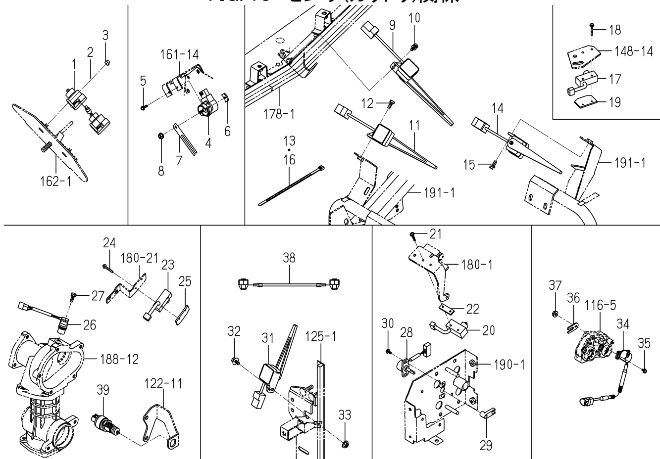
FIG. 78 センサ(カリトリ)関係
