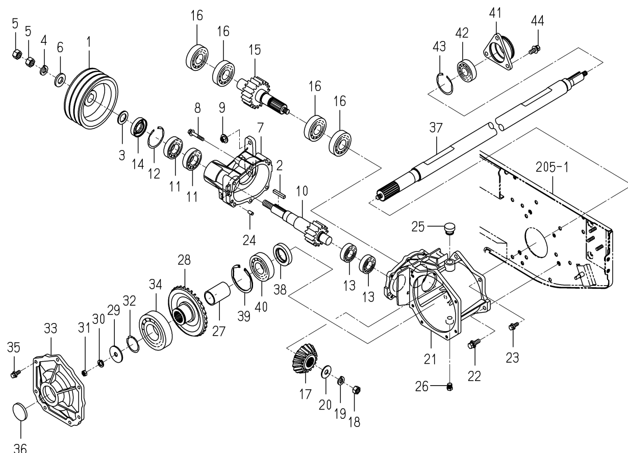
FIG.222 ドライブ(シリンダ)関係
