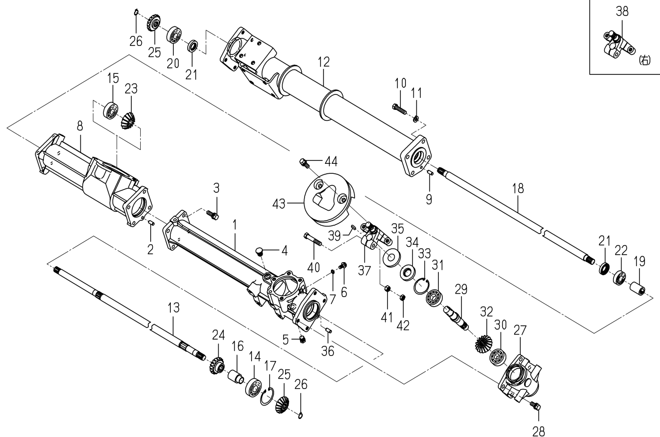
FIG.186 ケース(ギヤ／ロー)関係
