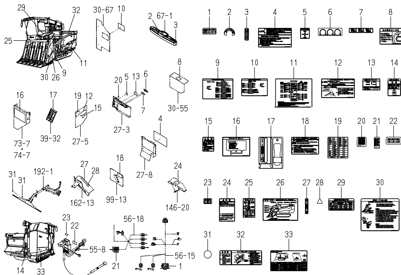
FIG.275 ラベル(コントロール, コーシヨン)(ZC型除く)(図1/2)
