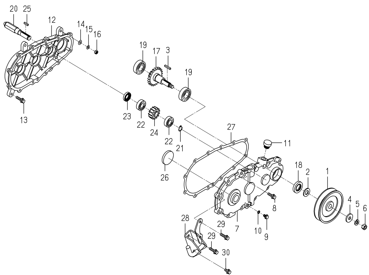
FIG.224 ドライブ(エジェクタ)関係(T型)
