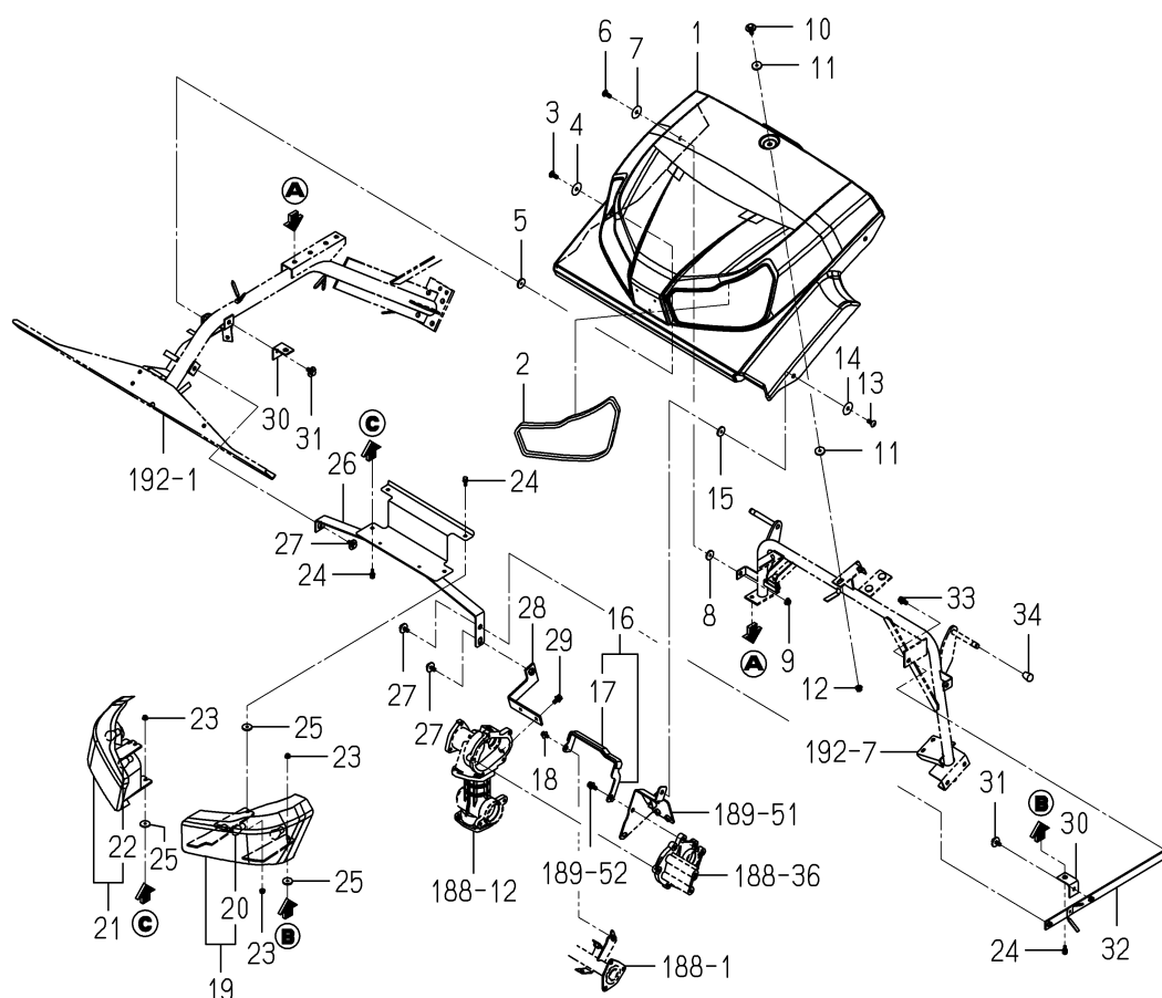
FIG.198 カバー(ダスト)関係(ZC型)
