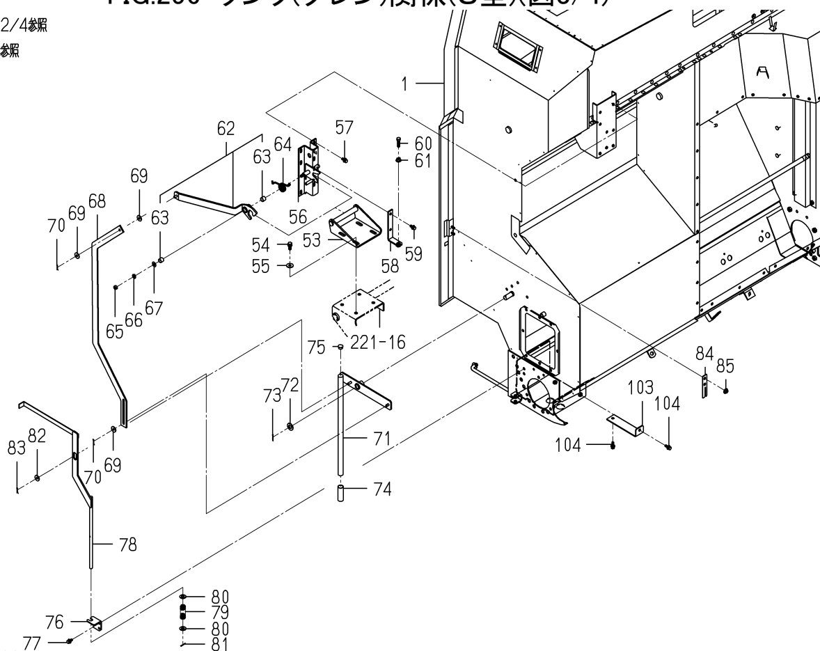
FIG.256 タンク(グレン)関係(S型)(図3/4)
