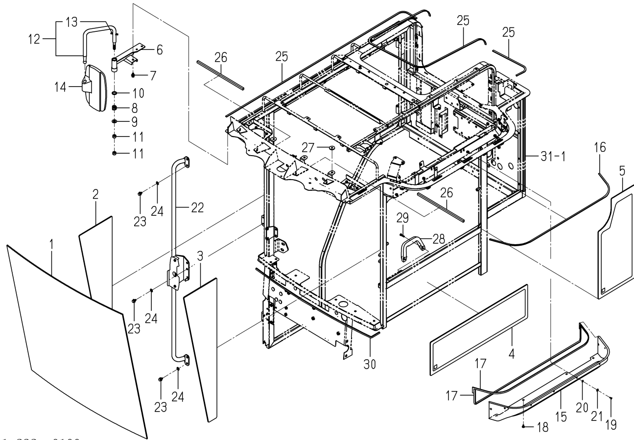
FIG. 43 ガラス(キャビン)関係(ZC型)
