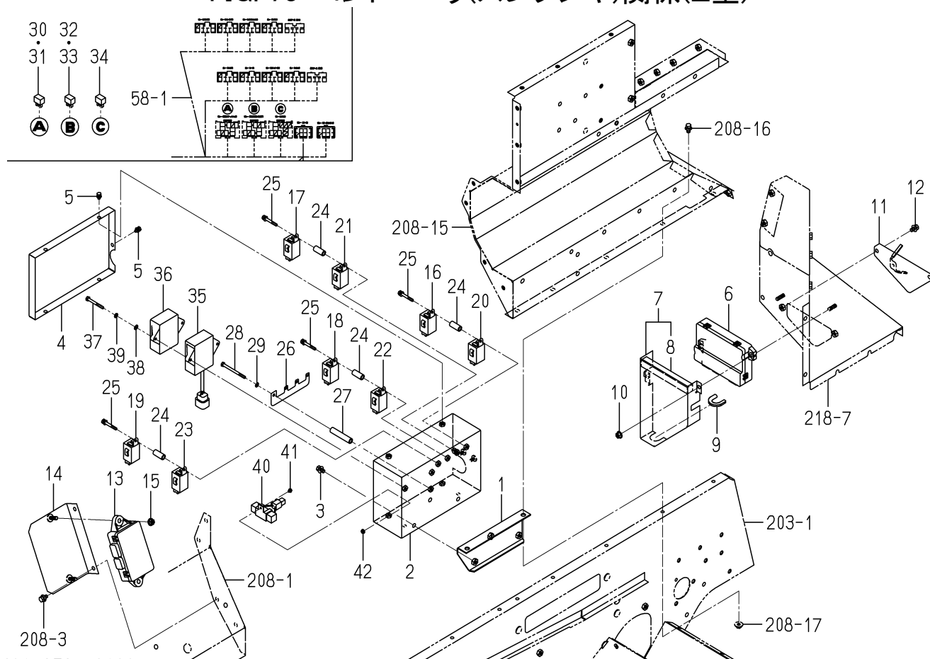
FIG. 73 コントローラ(スレッシヤ)関係(Z型)
