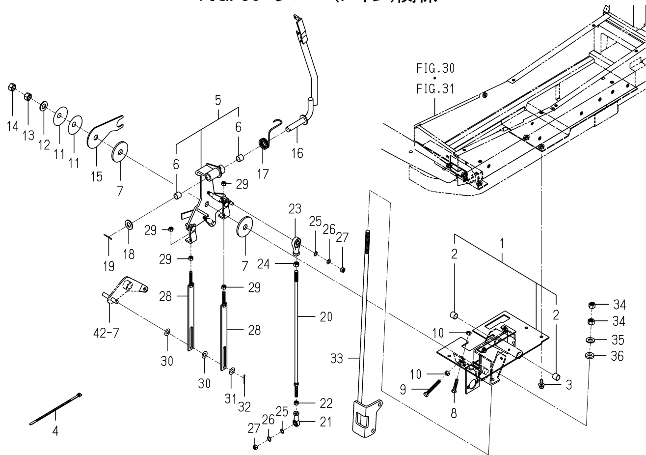
FIG. 36 レバー(メイン)関係
