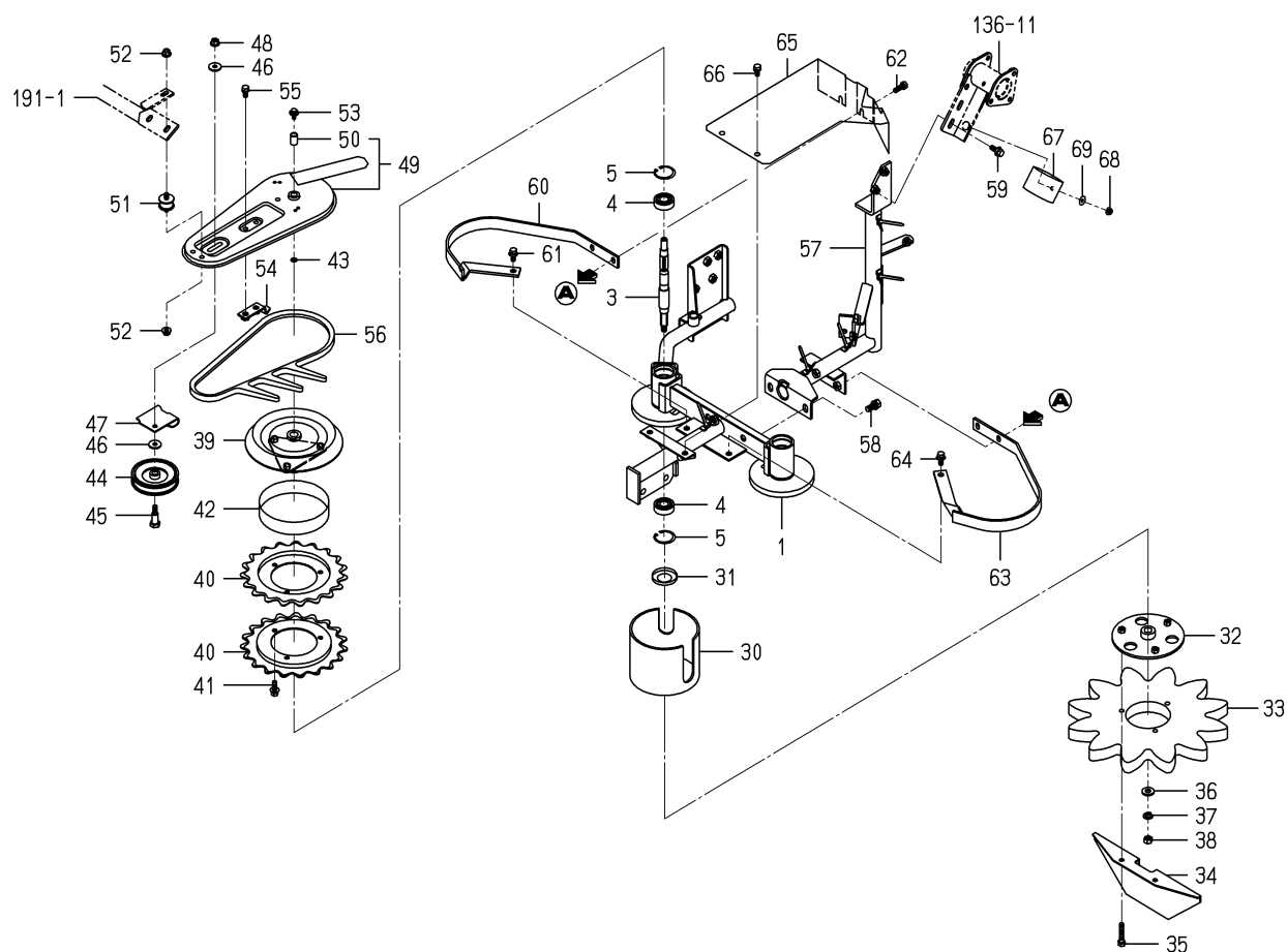
FIG.142 レイクアツプ(LH／2ND, 3RD)関係(図2/2)
