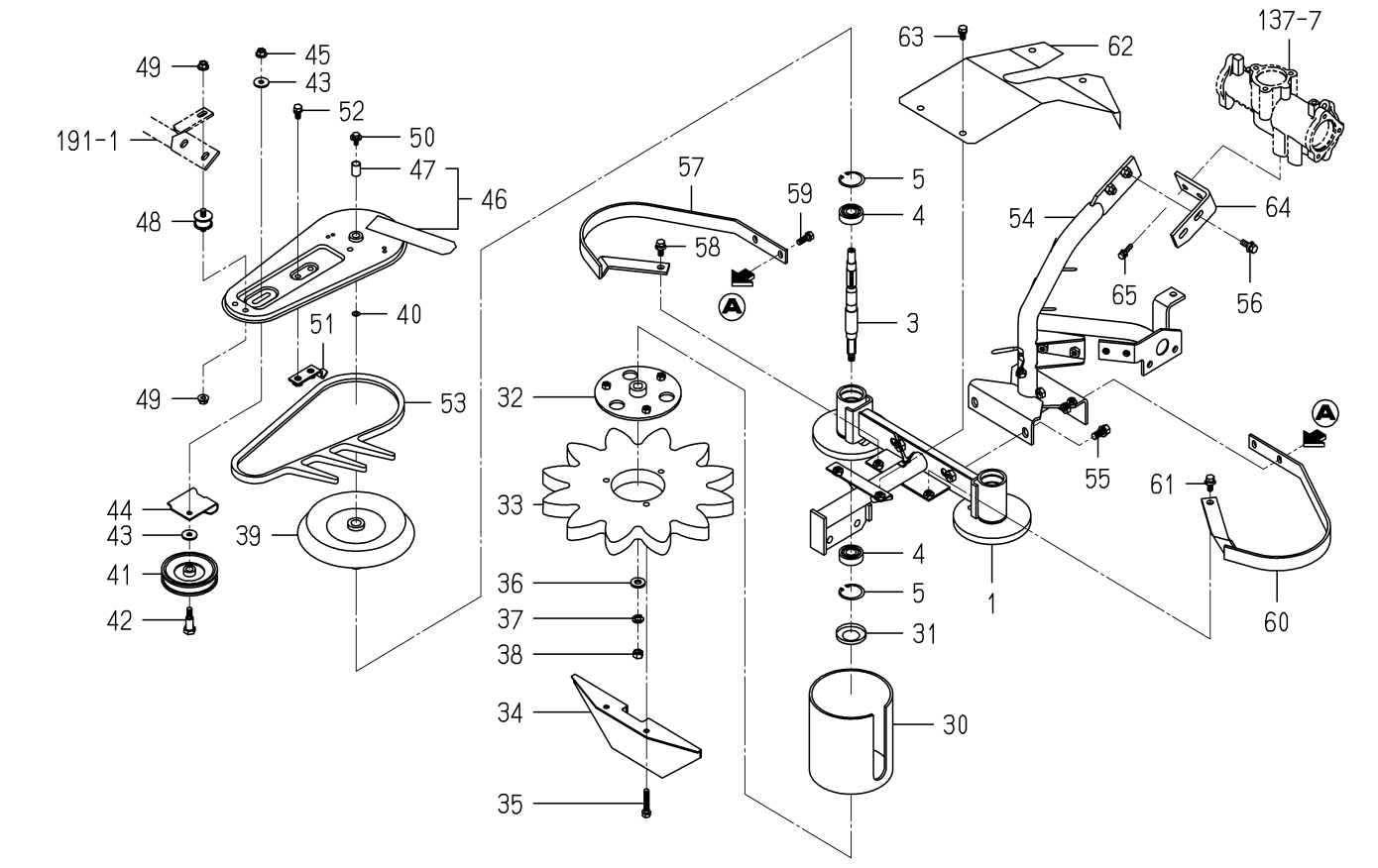
FIG.143 レイクアップ(RH／3RD, 2ND)関係(図2/2)
