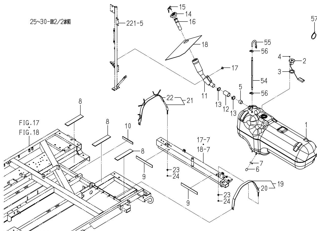
FIG. 89 タンク(フューエル)関係(図1/2)
