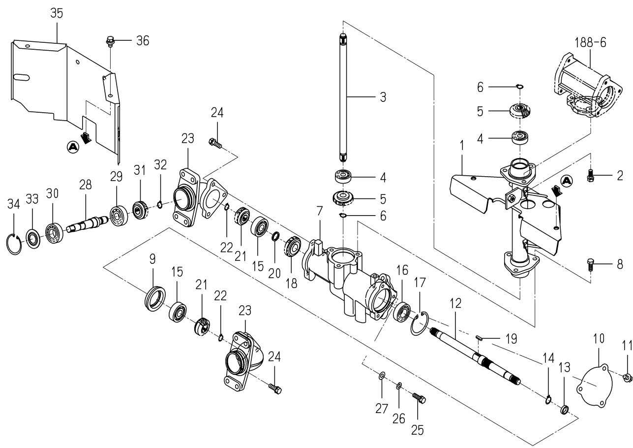
FIG.137 チューブ(ライズアップ/RH/3RD, 2ND)関係
