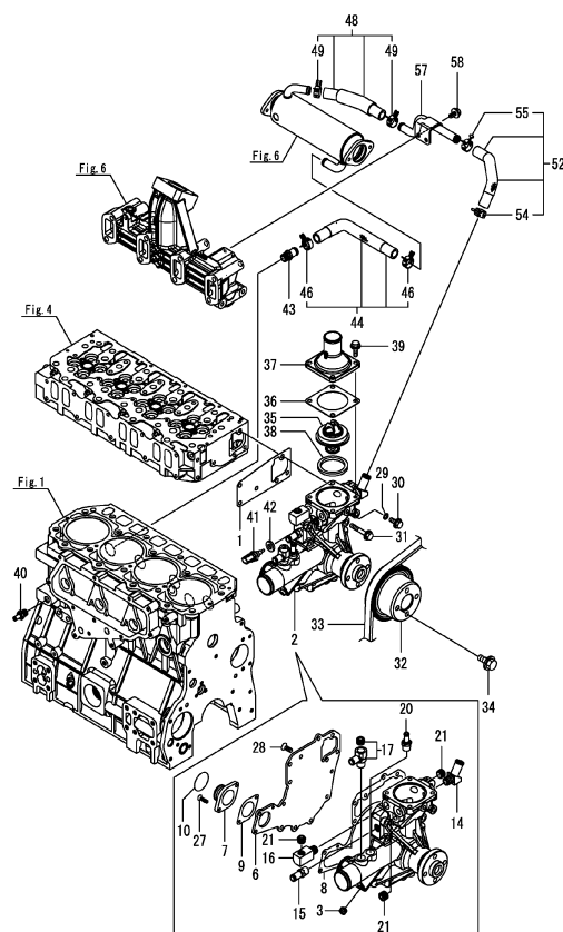
FIG.013 冷却水システム
