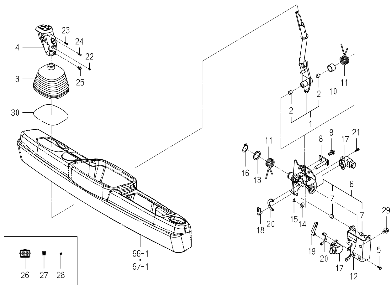
FIG. 38 レバー(ステアリング)関係
