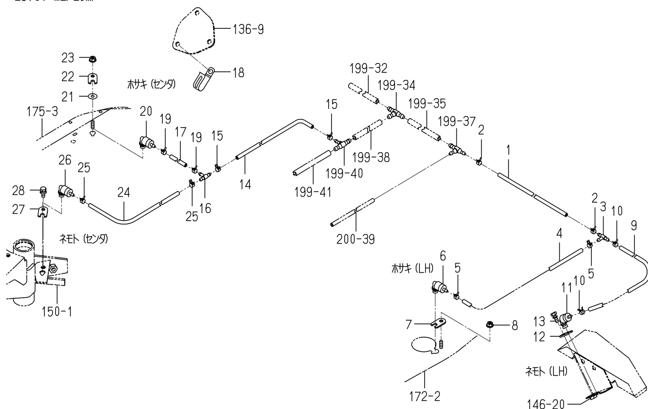
FIG.201 ノズル(オイリング／カリトリハンソウ)関係(図1/2)
