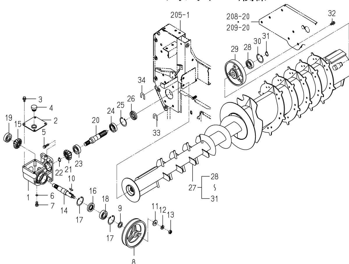
FIG.216 シリンダ(2ND)関係
