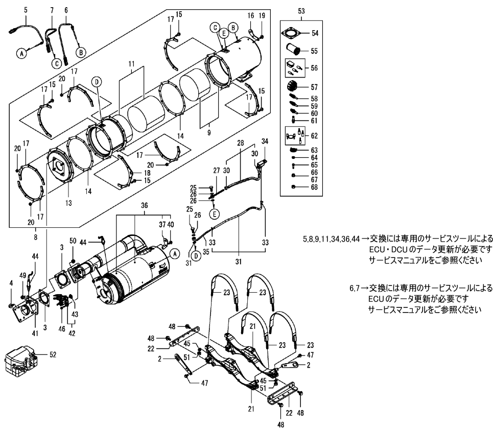
FIG.024 ATDユニット
