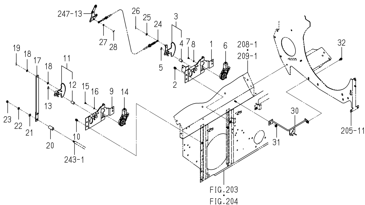
FIG.240 モータ(シーブ, ウインド)関係
