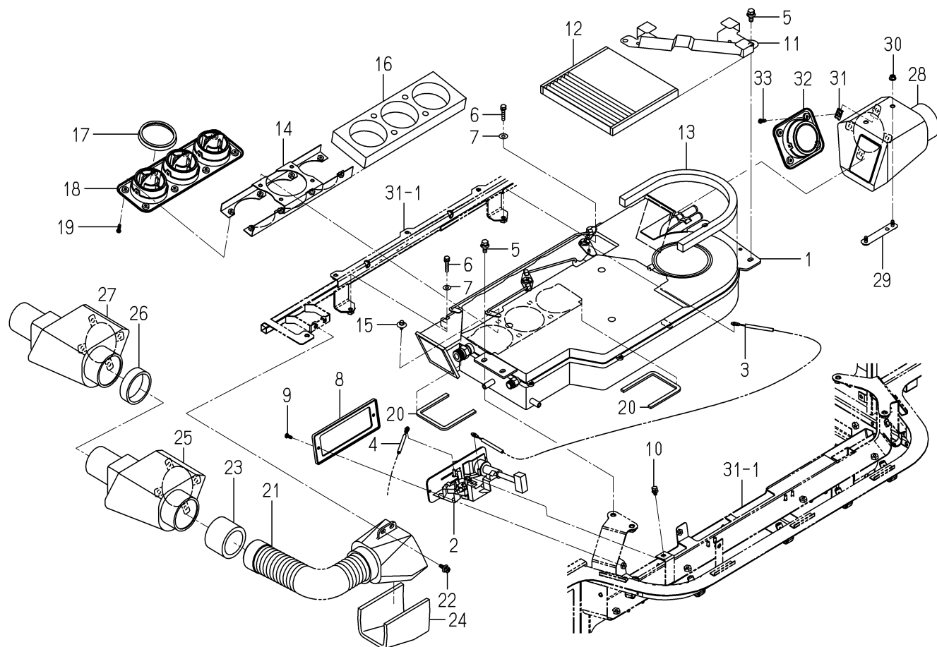
FIG. 53 エアコン(キャビン)関係(ZC型)(図1/3)
