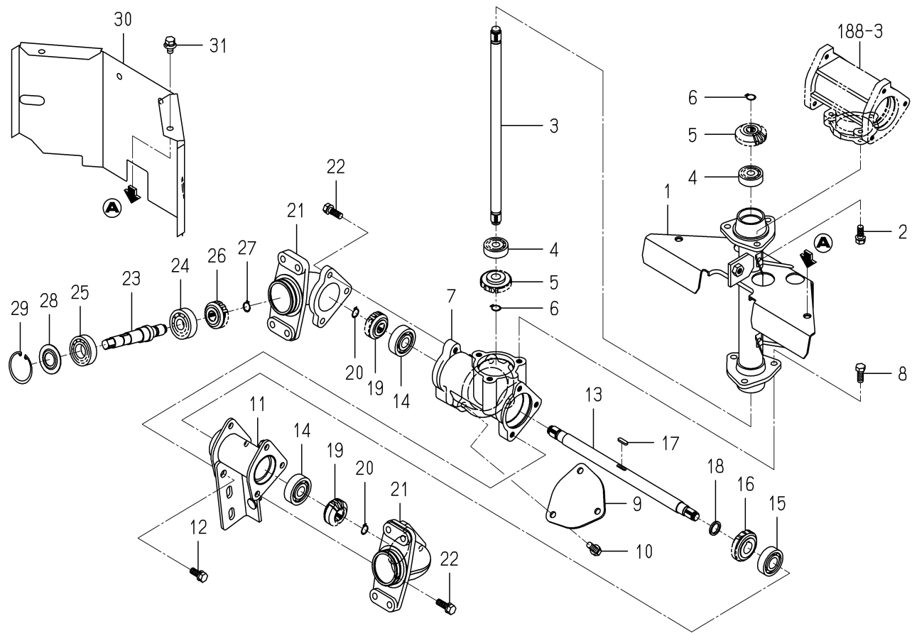
FIG.136 チューブ(ライズアップ/LH/2ND, 3RD)関係
