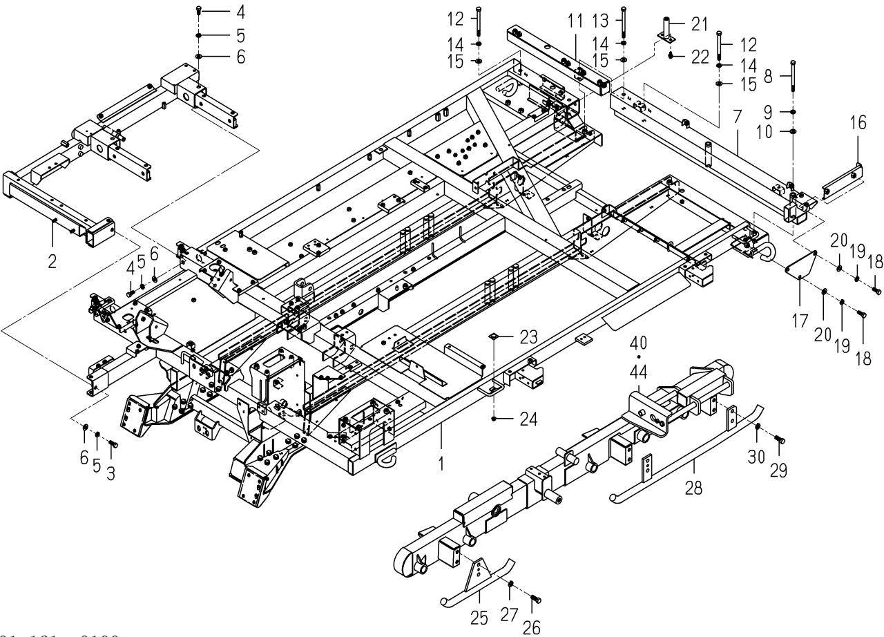
FIG. 17 フレーム(ソウコウ／オープン)関係(A型)(図1/2)
