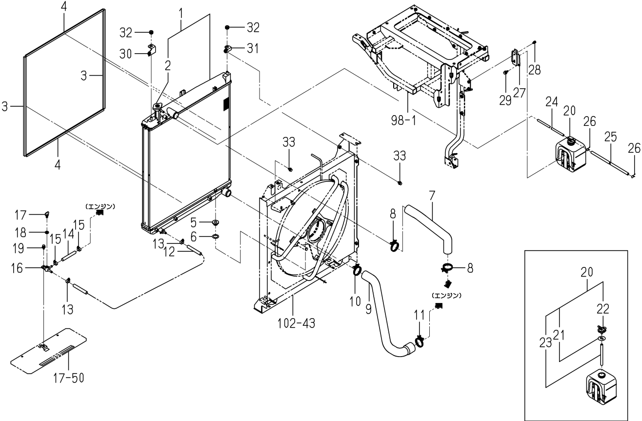
FIG. 92 ラジエータ関係(ZC型除く)(図1/2)
