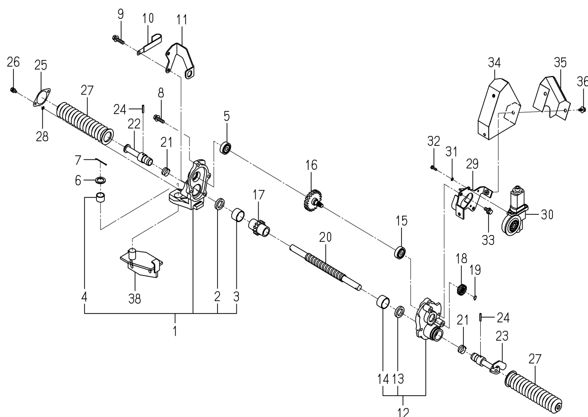
FIG.122 ガイド(ナロー／LH)関係(図1/2)
