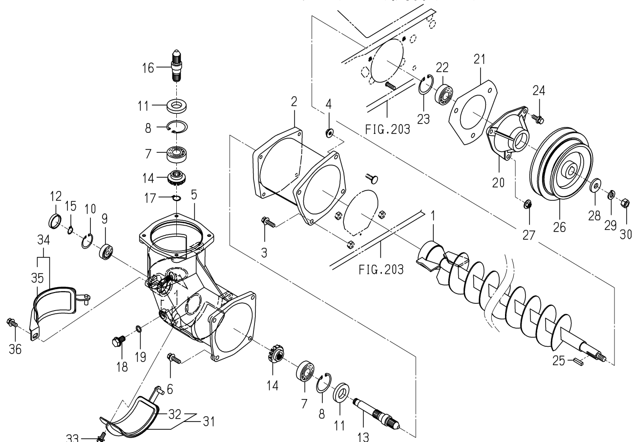
FIG.248 スパイラル(1ST)関係(Z型)
