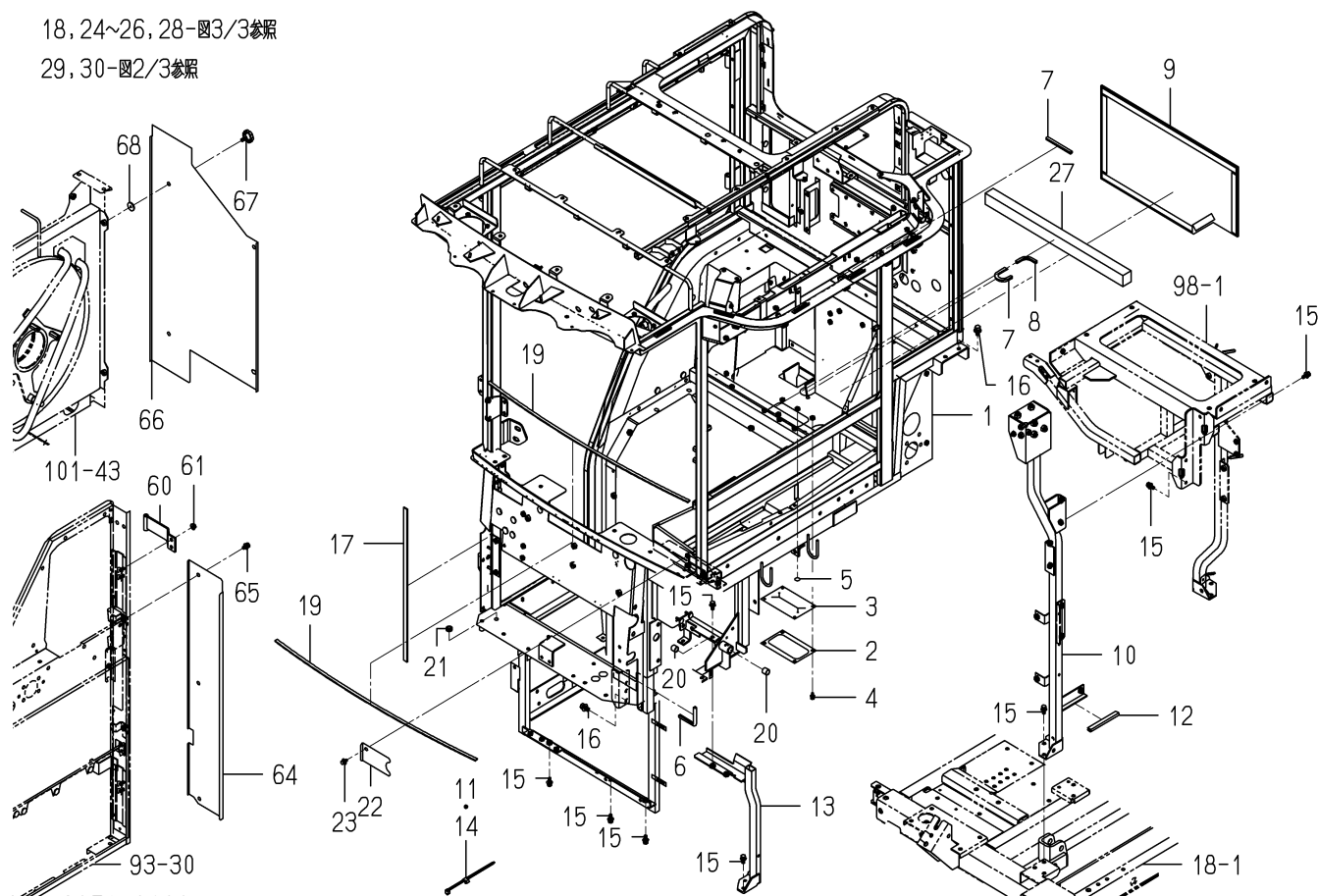
FIG. 31 フレーム(コントロール)関係(ZC型)(図1/3)
