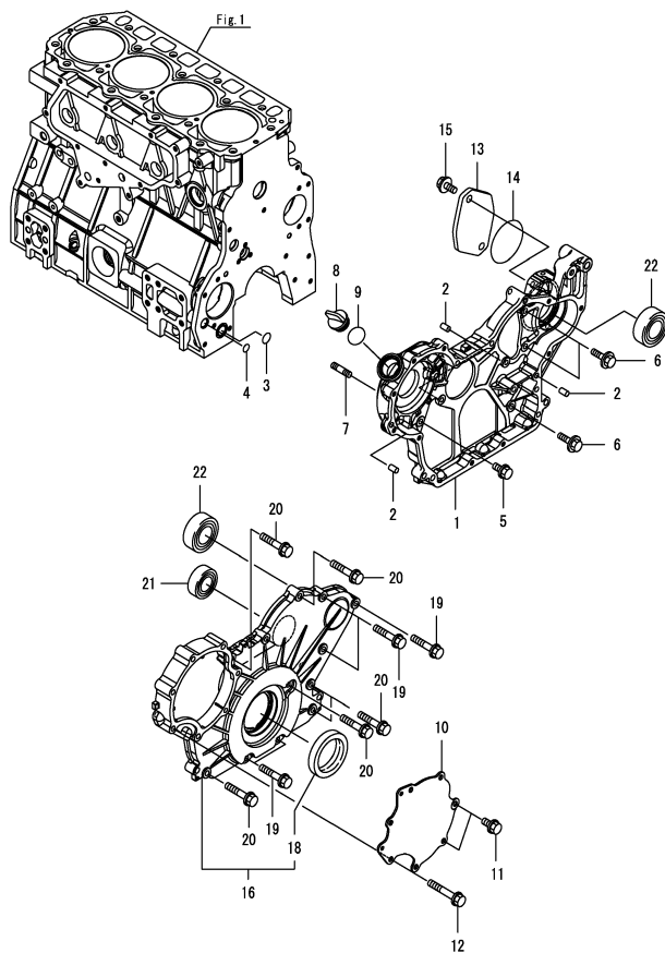
FIG.002 ギヤケース
