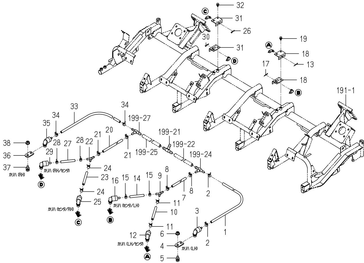
FIG.200 ノズル(オイリング／ヒキオコシ、カリハ)関係(図1/2)
