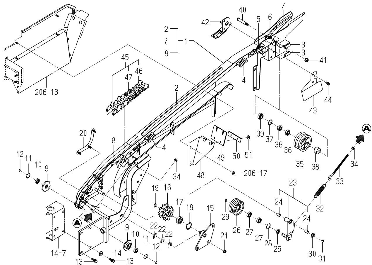
FIG.230 チェン(フイード)関係
