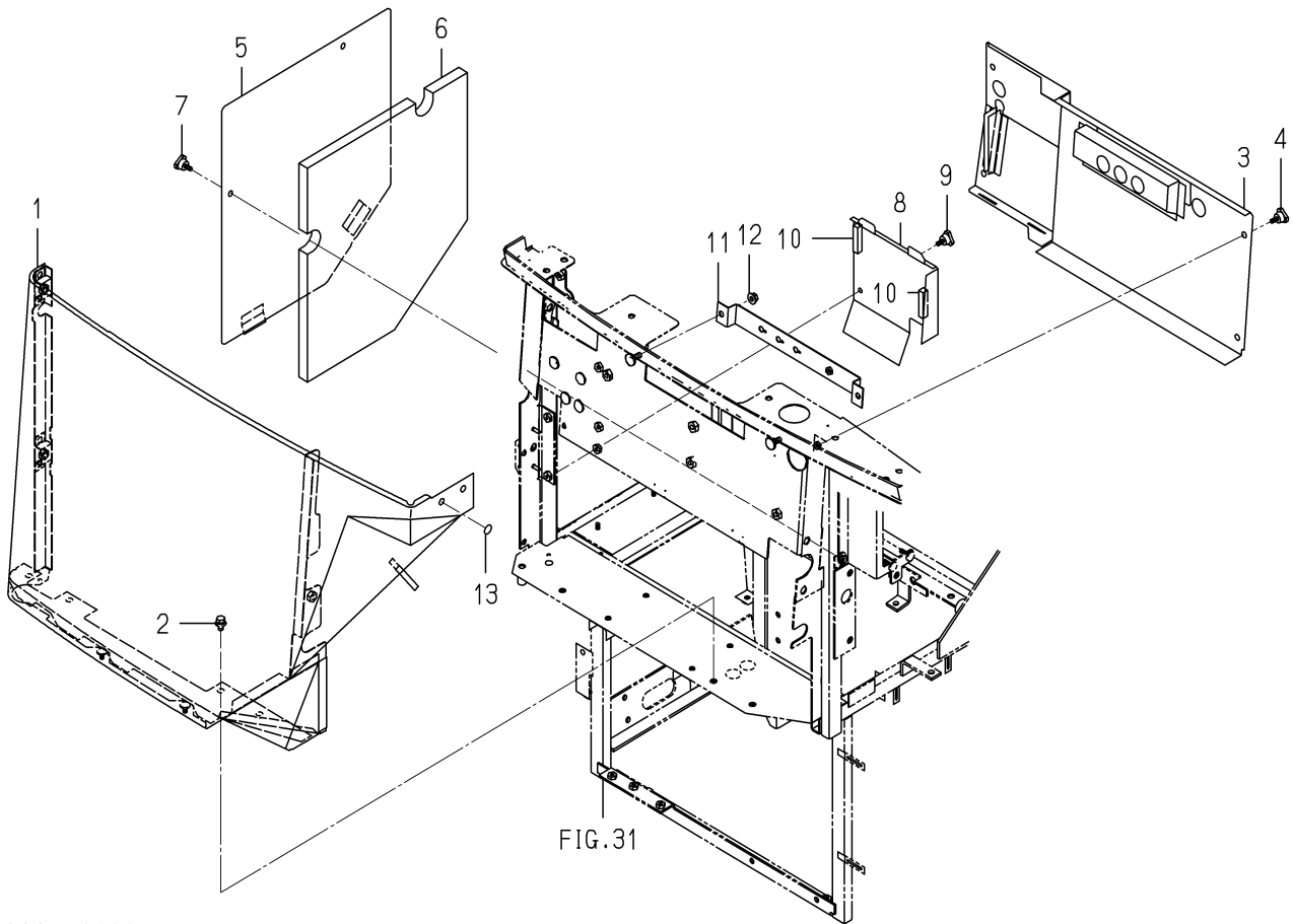
FIG. 28 カバー(コントロール)関係(ZC型)
