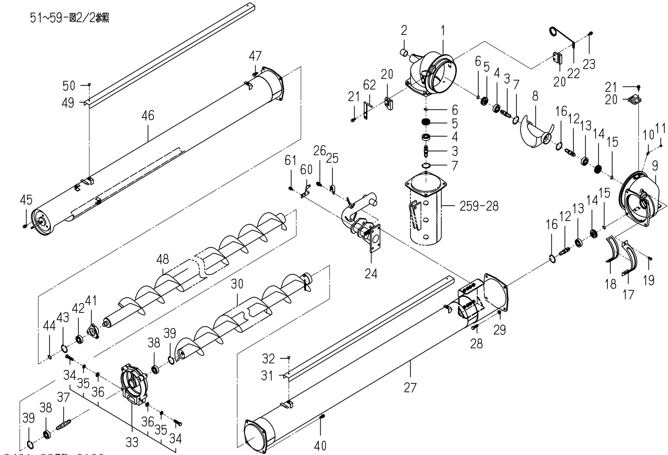
FIG.261 オーガ(アツパ)関係(T型)(図1/2)
