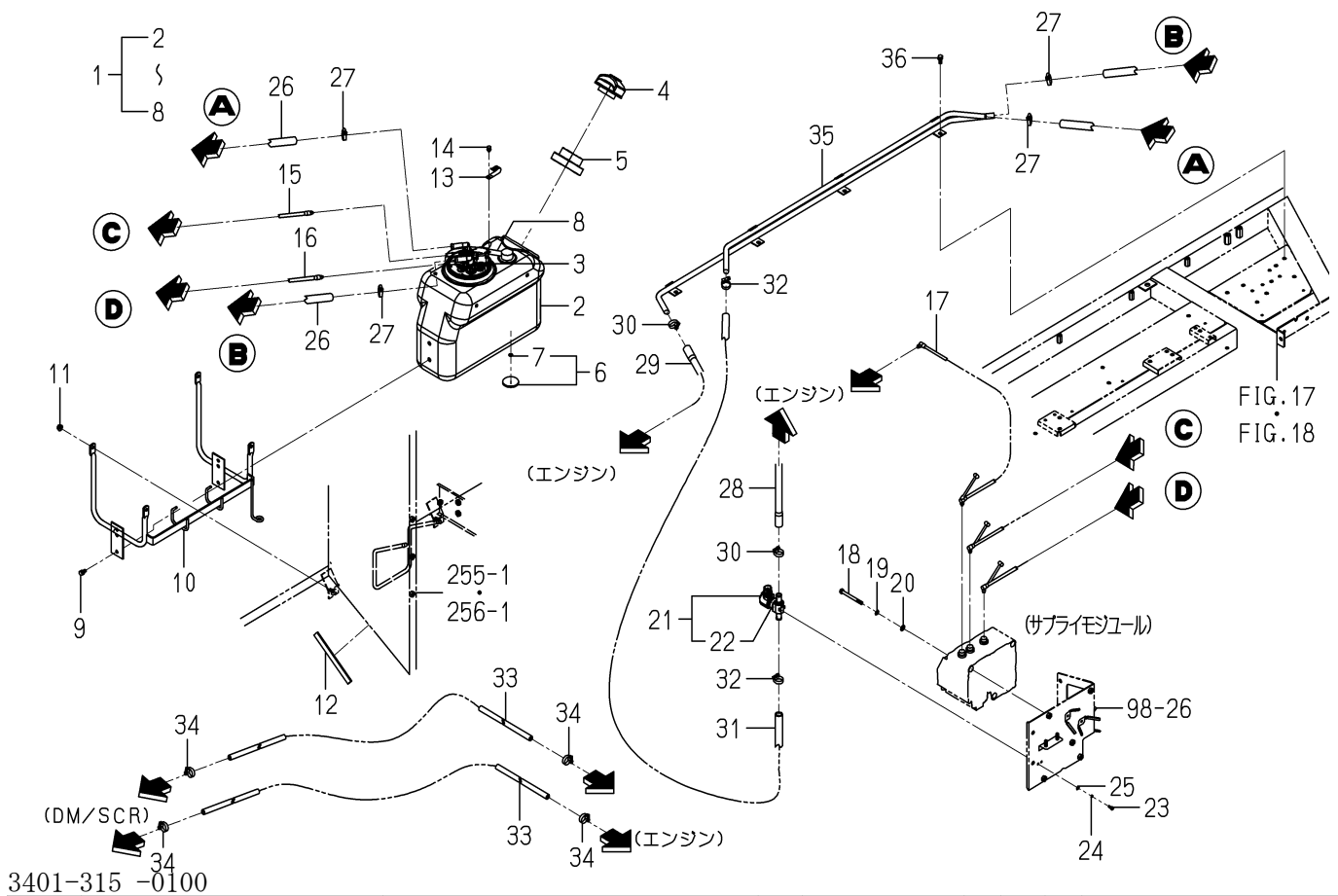
FIG. 91 タンク(DEF)関係
