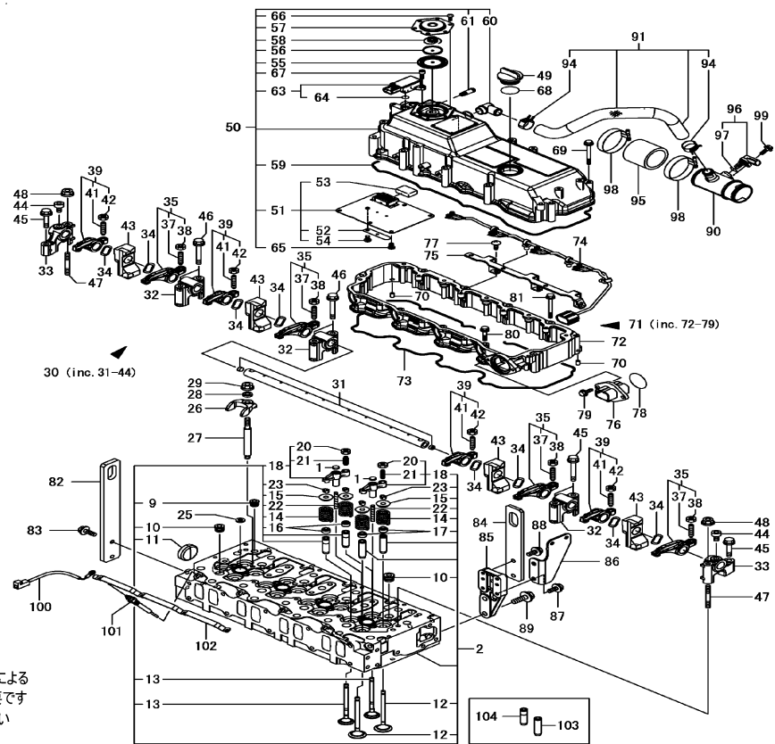
FIG.004 シリンダヘッド&ボンネット
