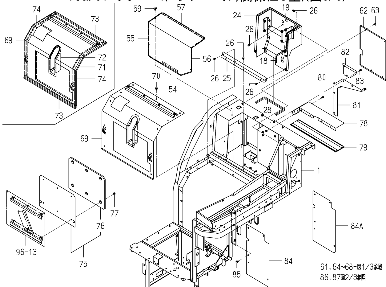
FIG. 31 フレーム(コントロール)関係(ZC型)(図3/3)
