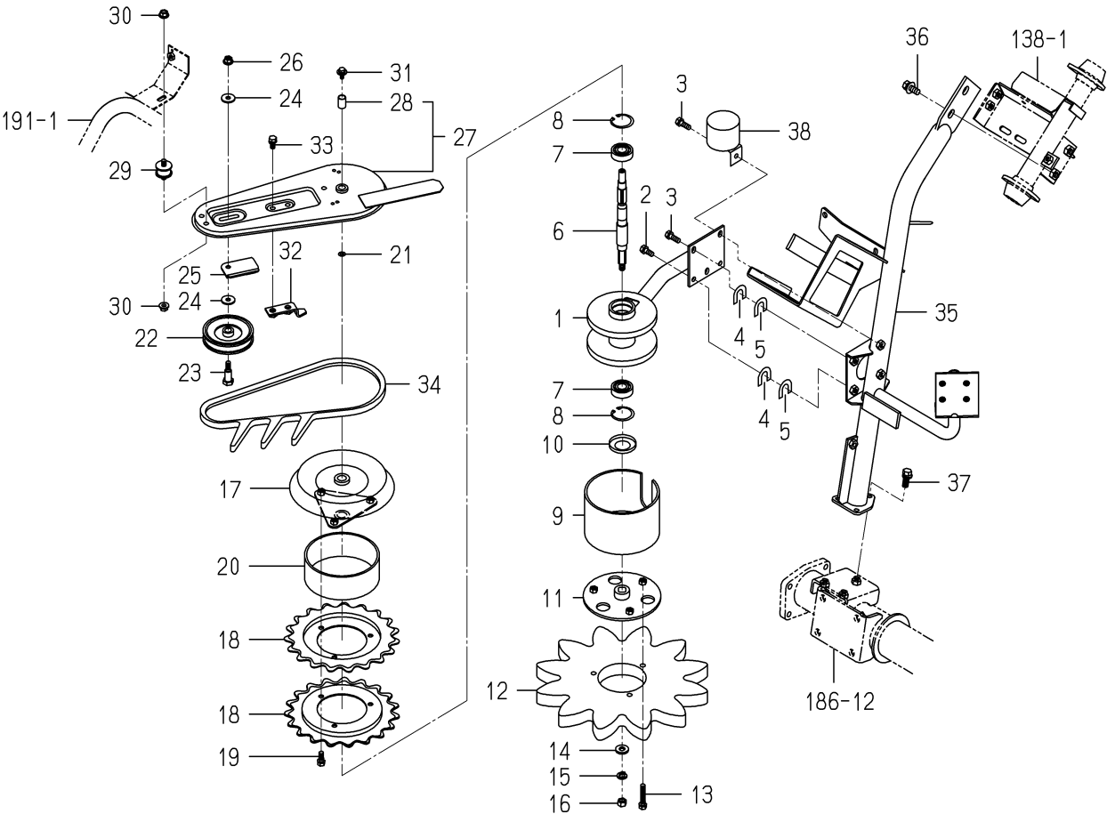
FIG.144 レイクアップ(RH／1ST)関係
