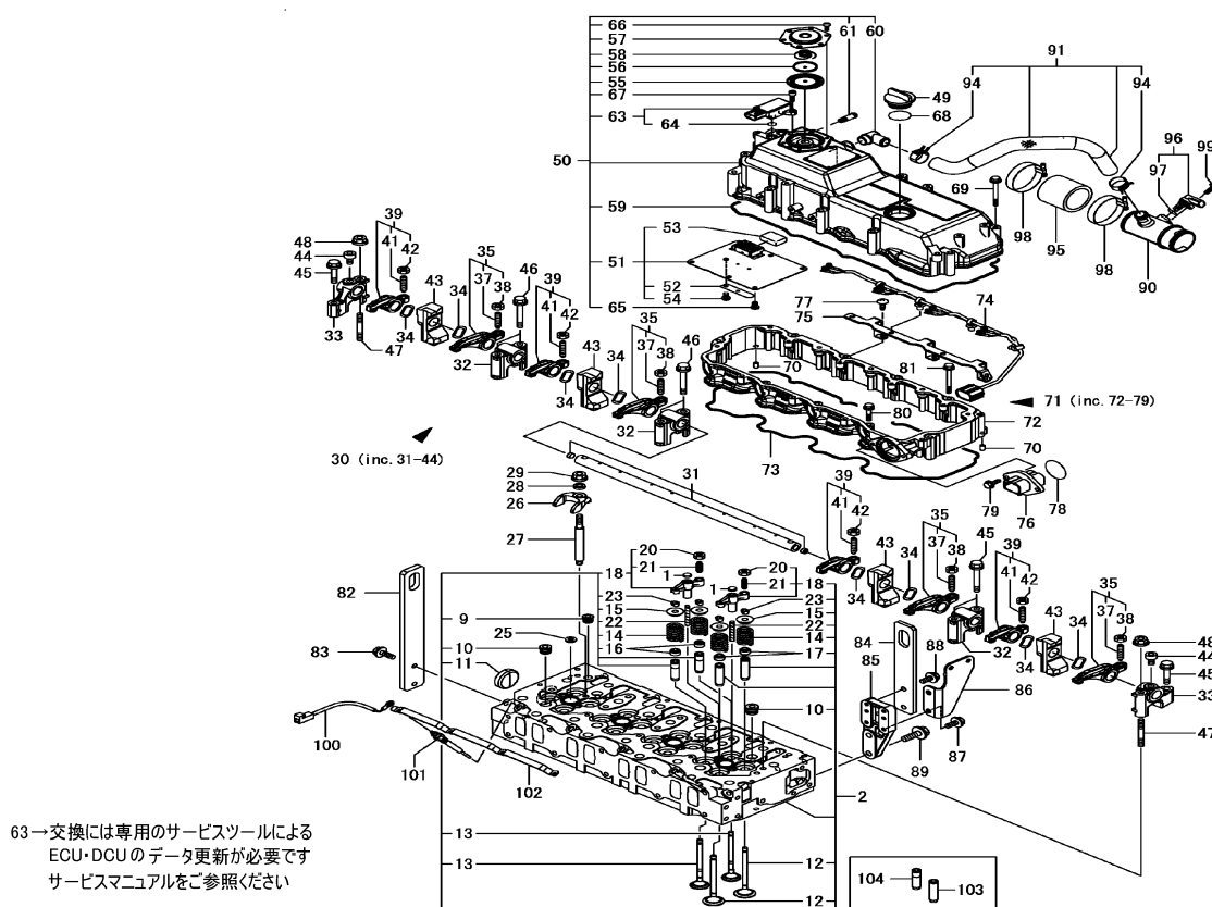
FIG.004 シリンダヘッド&amp;ボンネット
